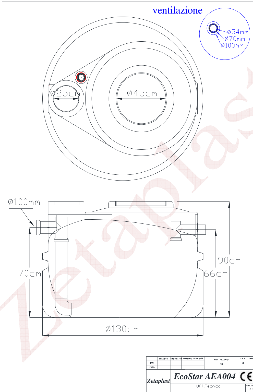
Fig.7 – Schema tecnico
