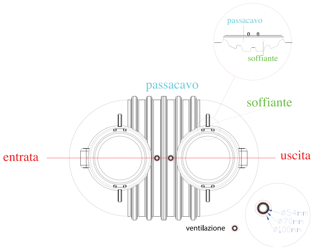
Fig.2 – Posizionamento collegamenti biogas-ventilazione, soffiante e ricircolo
