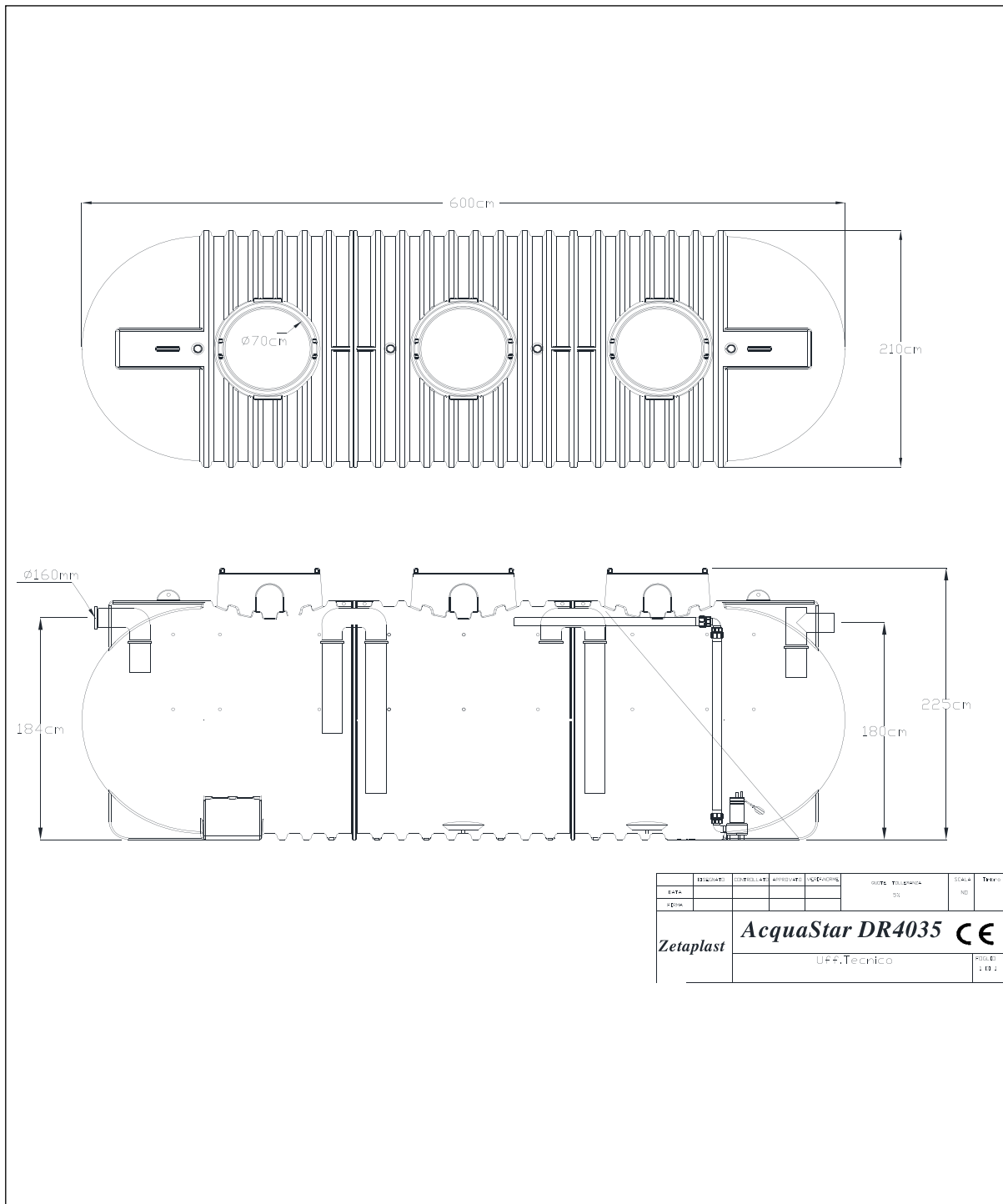
Fig.6 – Schema tecnico
