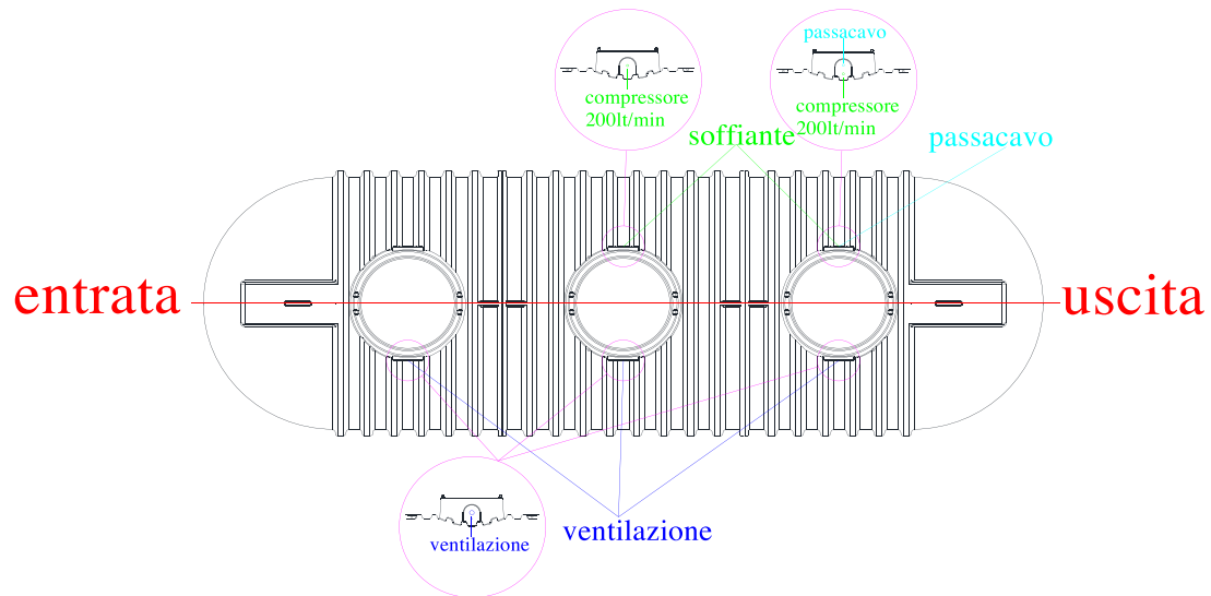
Fig.2 – Posizionamento collegamenti biogas-ventilazione, soffiante e ricircolo
