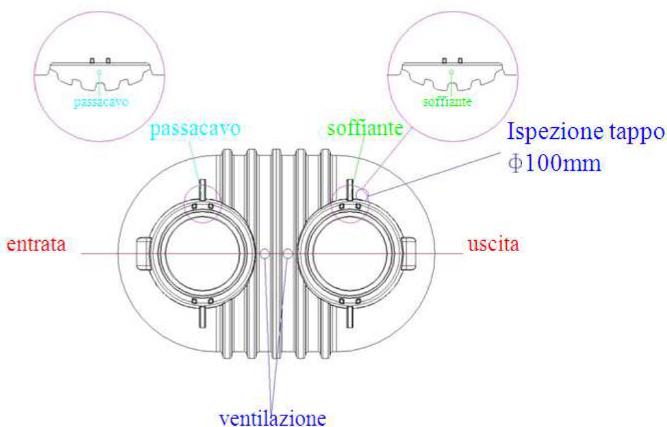
Fig.2 – Posizionamento collegamenti biogas, ossigenazione e pompa
