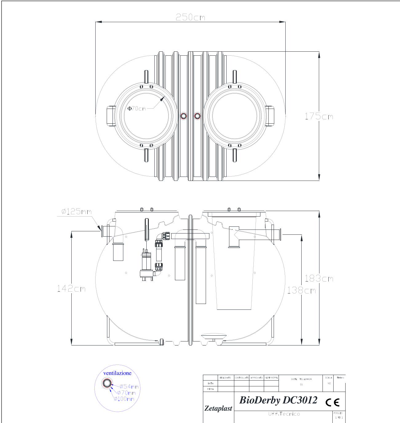
Fig.6 – Schema tecnico
