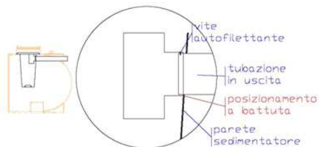
Installazione sedimentatore
