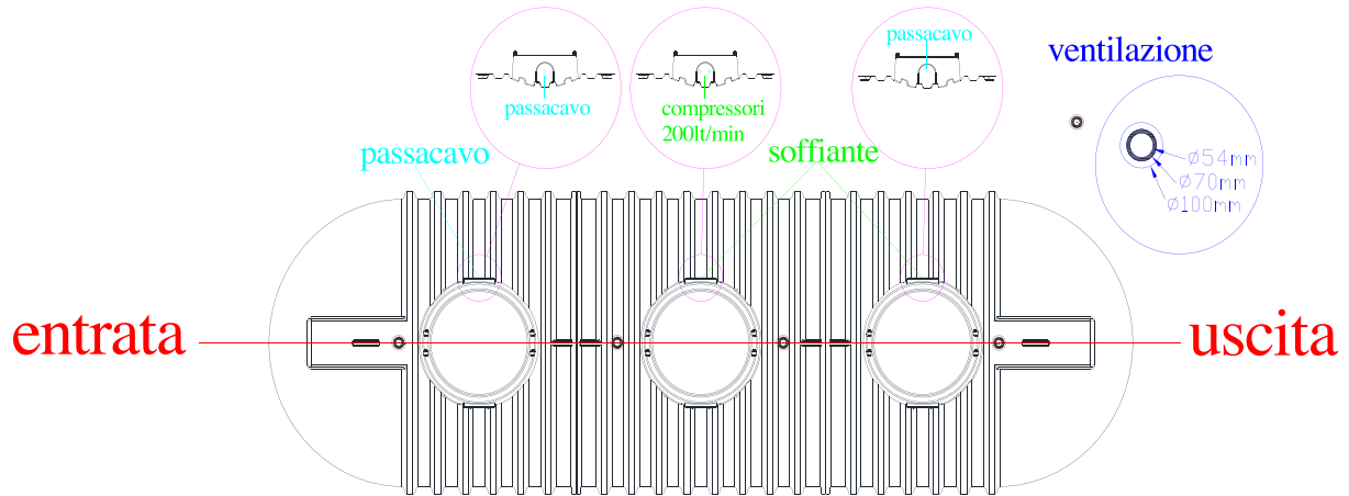
Fig.2 – Posizionamento collegamenti biogas, ossigenazione e pompa
