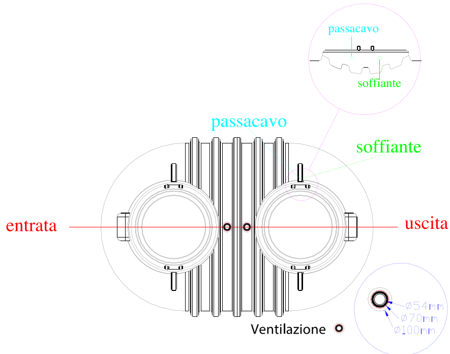
Fig.2 – Posizionamento collegamenti biogas-ventilazione, soffiante e ricircolo
