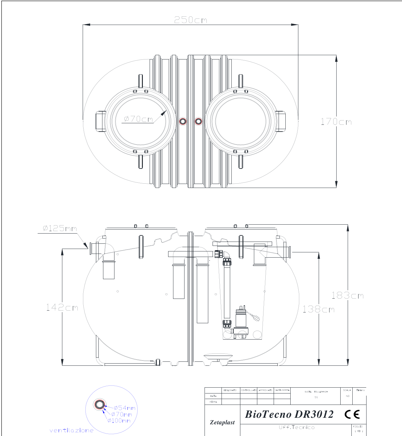
Fig.6 – Schema tecnico
