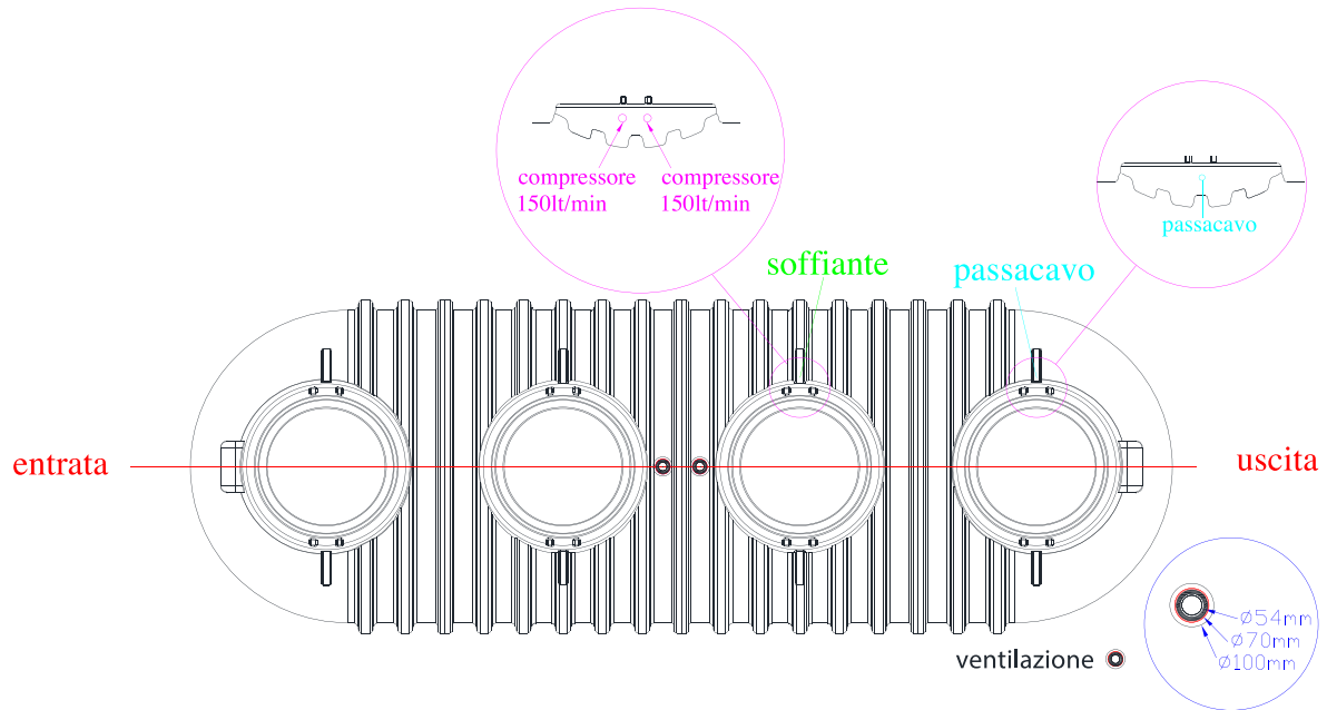
Fig.2 – Posizionamento collegamenti biogas-ventilazione, soffiante
