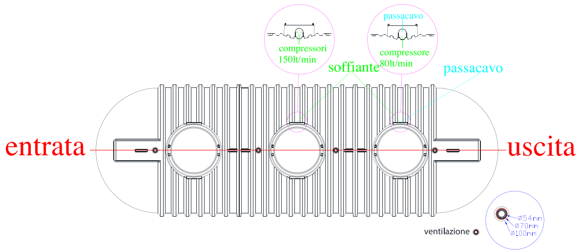
Fig.2 – Posizionamento collegamenti biogas-ventilazione, soffiante e ricircolo
