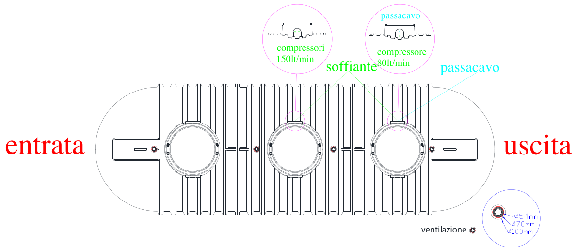
Fig.2 – Posizionamento collegamenti biogas-ventilazione, soffiante
