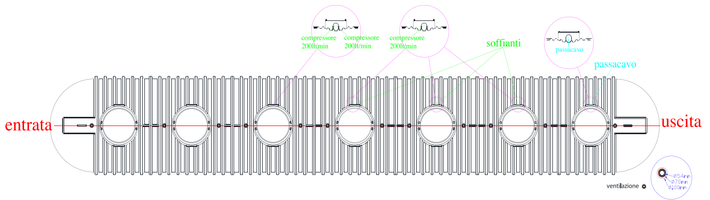
Fig.2 – Posizionamento collegamenti biogas-ventilazione, soffiante
