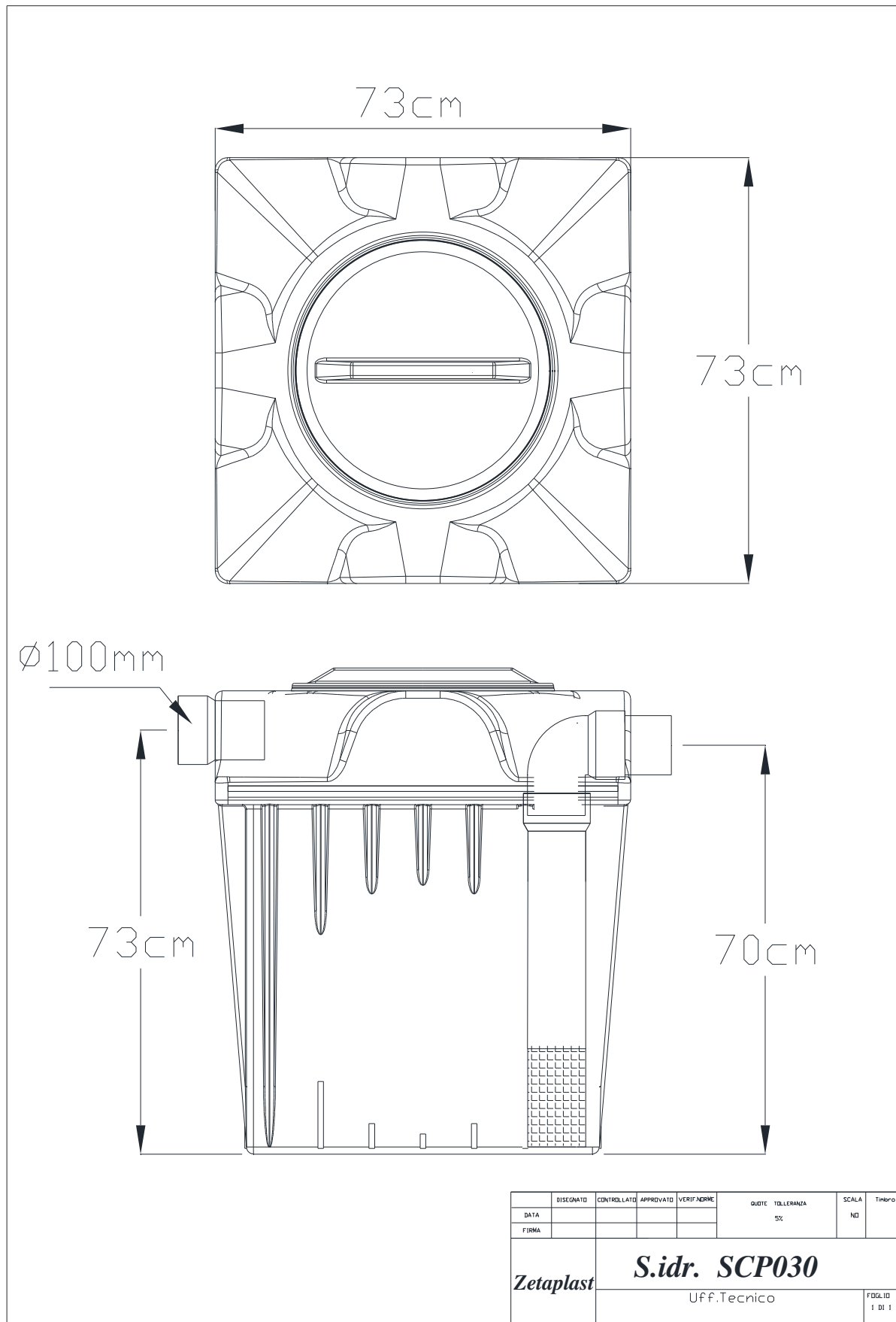
Fig.2 – Schema tecnico
