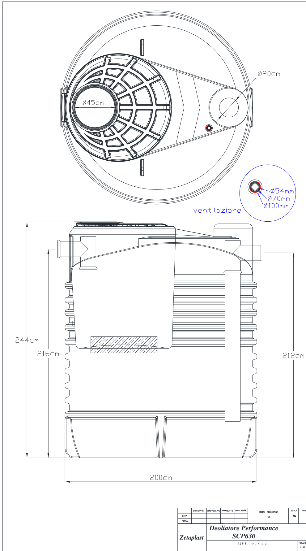
Fig.2 – Schema tecnico
