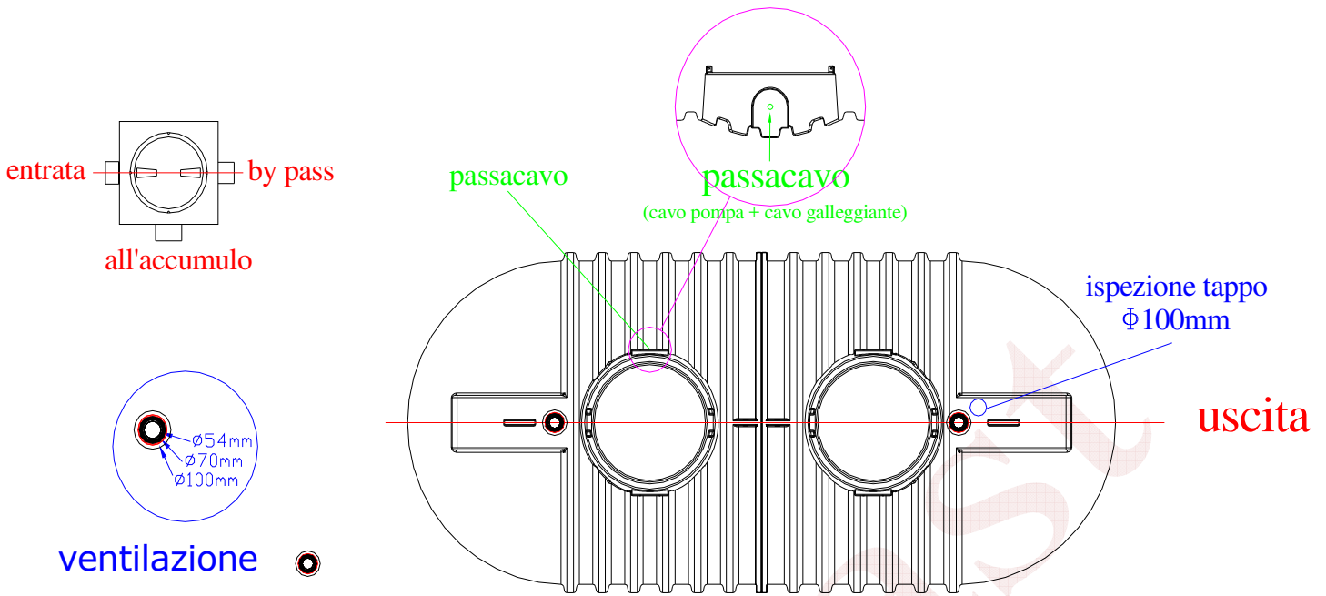
Fig.2 - Posizionamento collegamenti sfiati, cavo pompa e galleggiante
