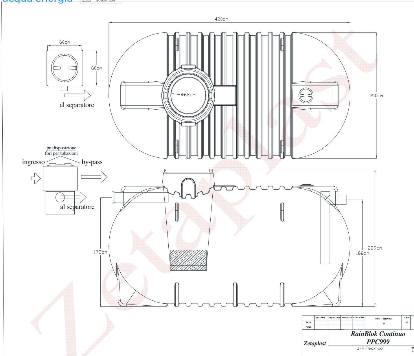
Fig. 3 – Schema tecnico
