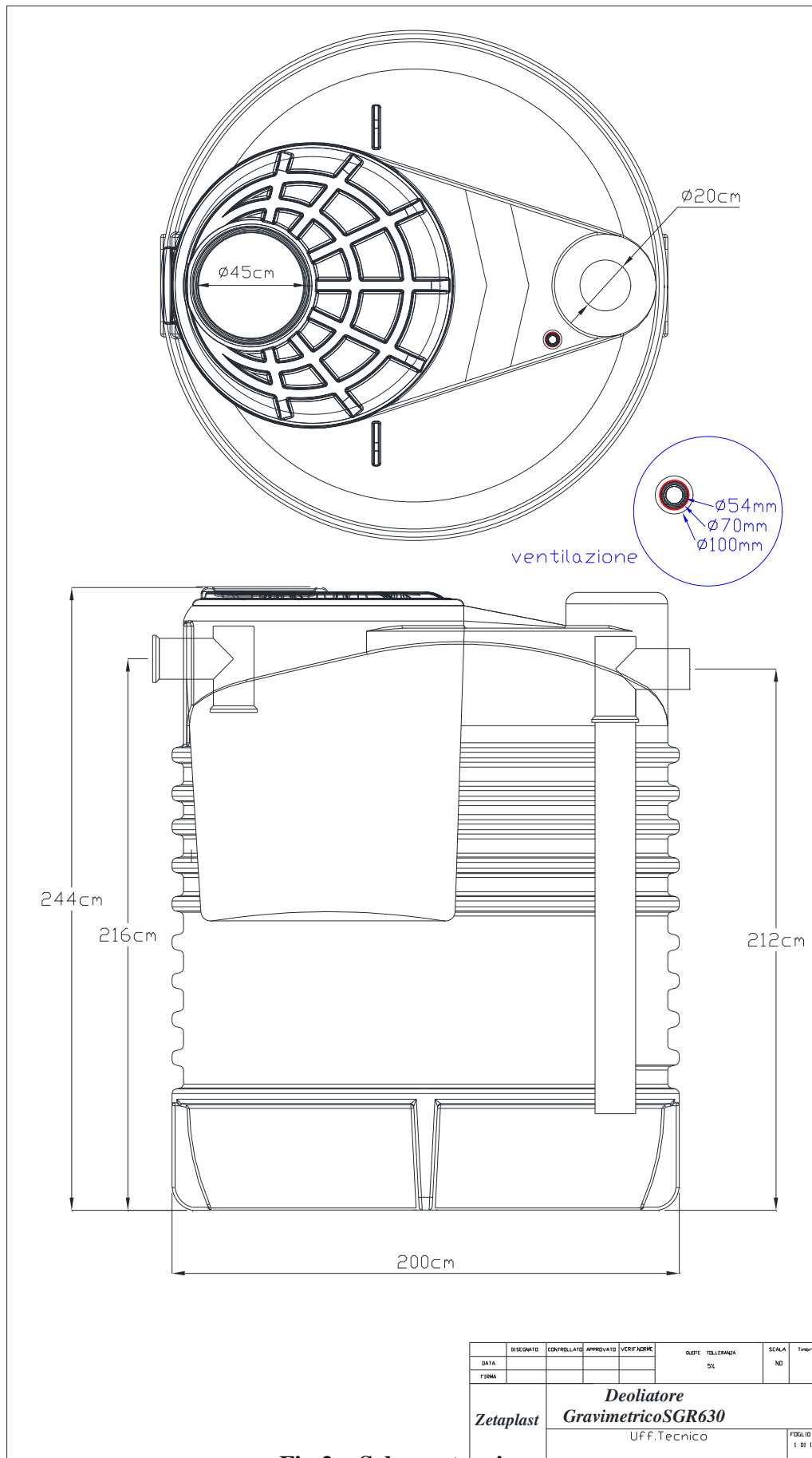
Fig.2 – Schema tecnico
