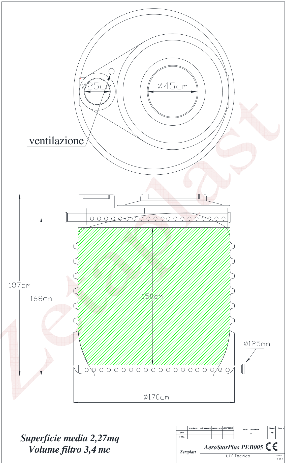
Fig.2 – Schema tecnico
