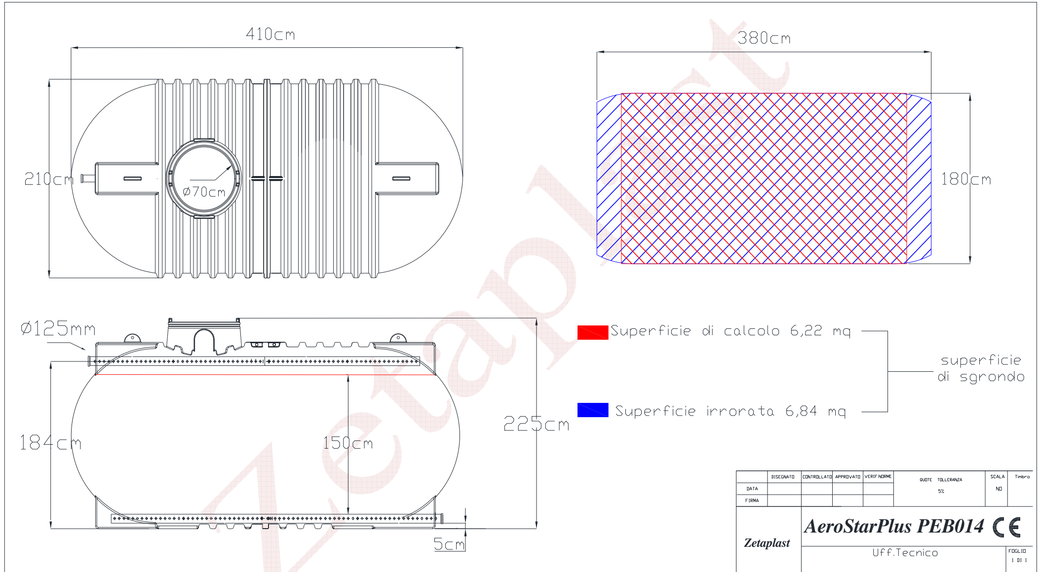
Fig.2 – Schema tecnico
