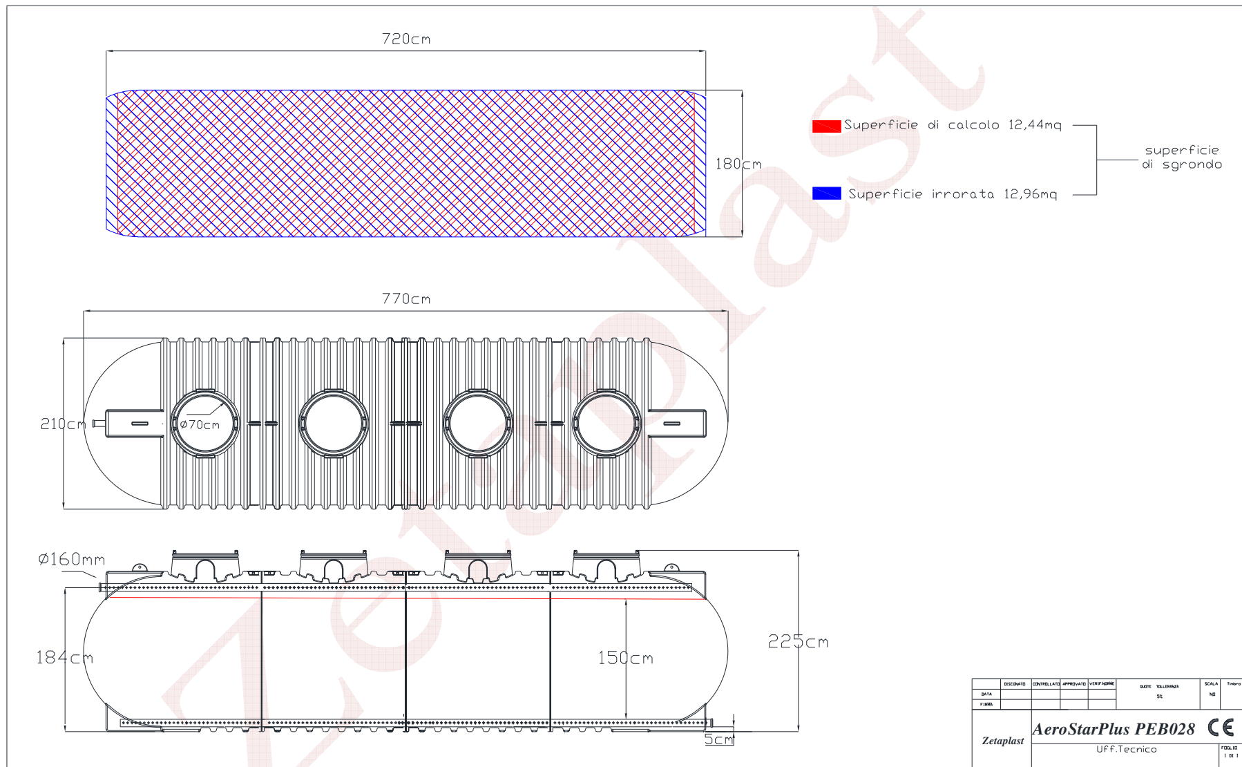
Fig.2 – Schema tecnico
