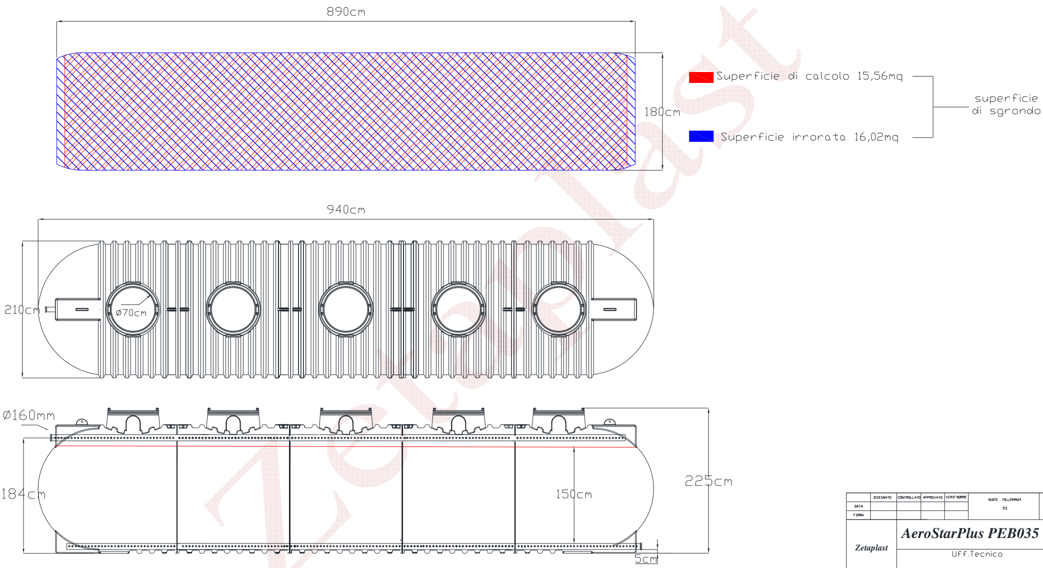
Fig.2 – Schema tecnico
