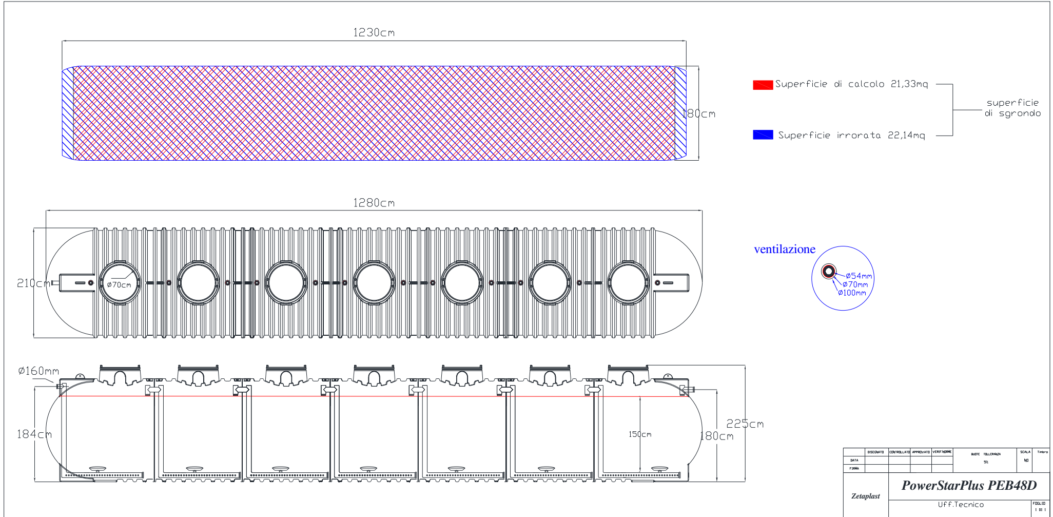
Fig.3 – Schema tecnico
