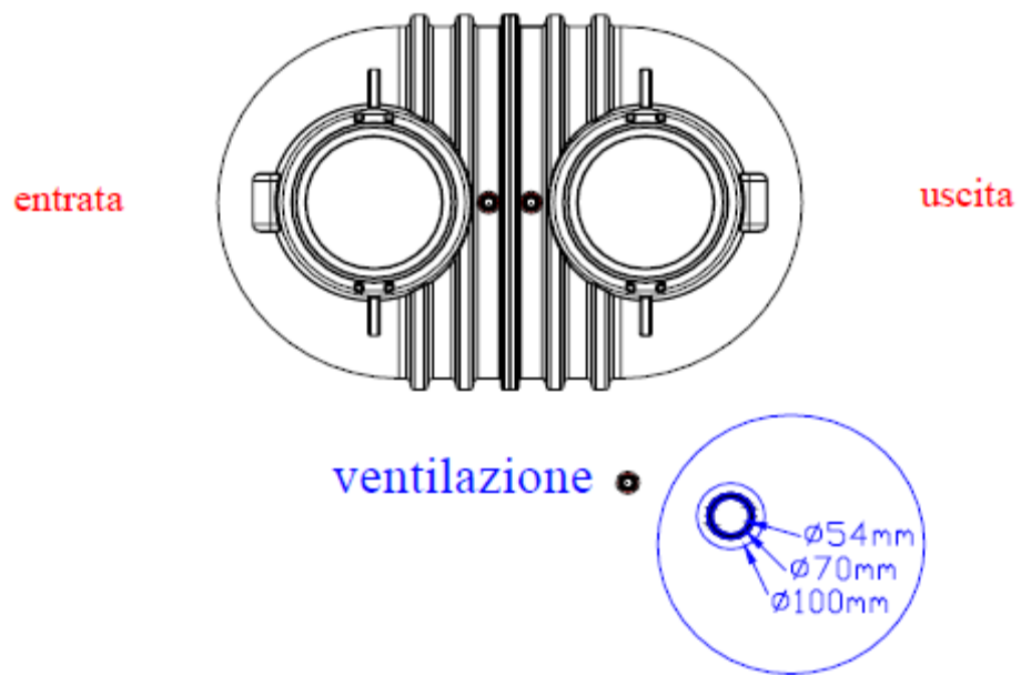
Fig.2 – Posizionamento collegamenti biogas
