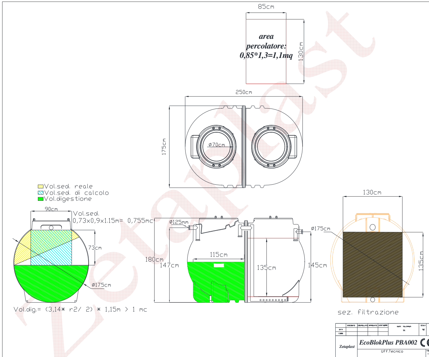
Fig.3 – Schema tecnico
