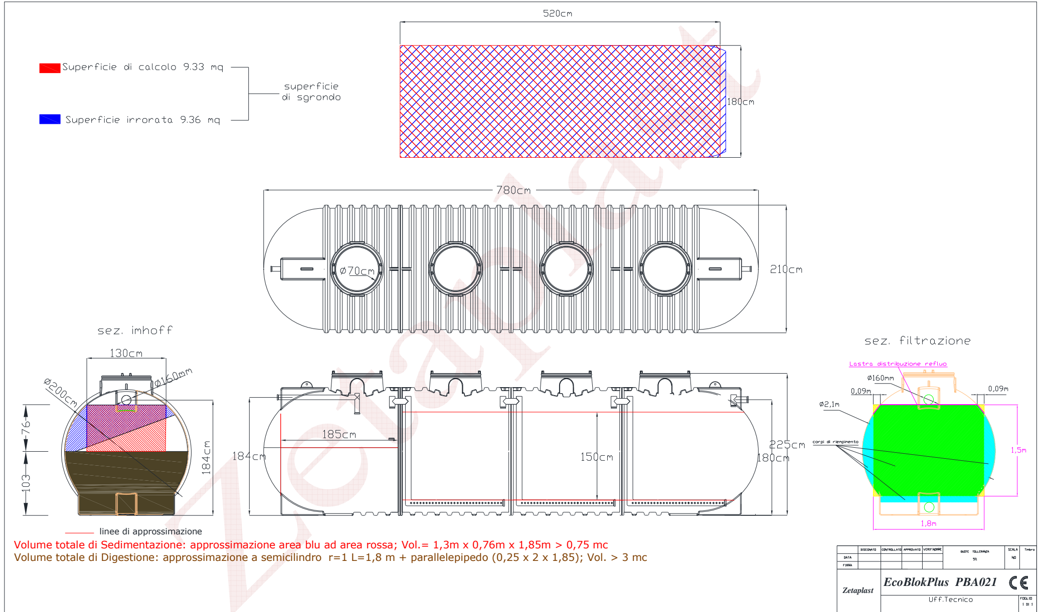
Fig.3 – Schema tecnico
