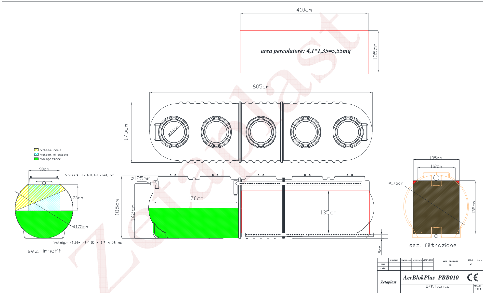
Fig.3 – Schema tecnico
