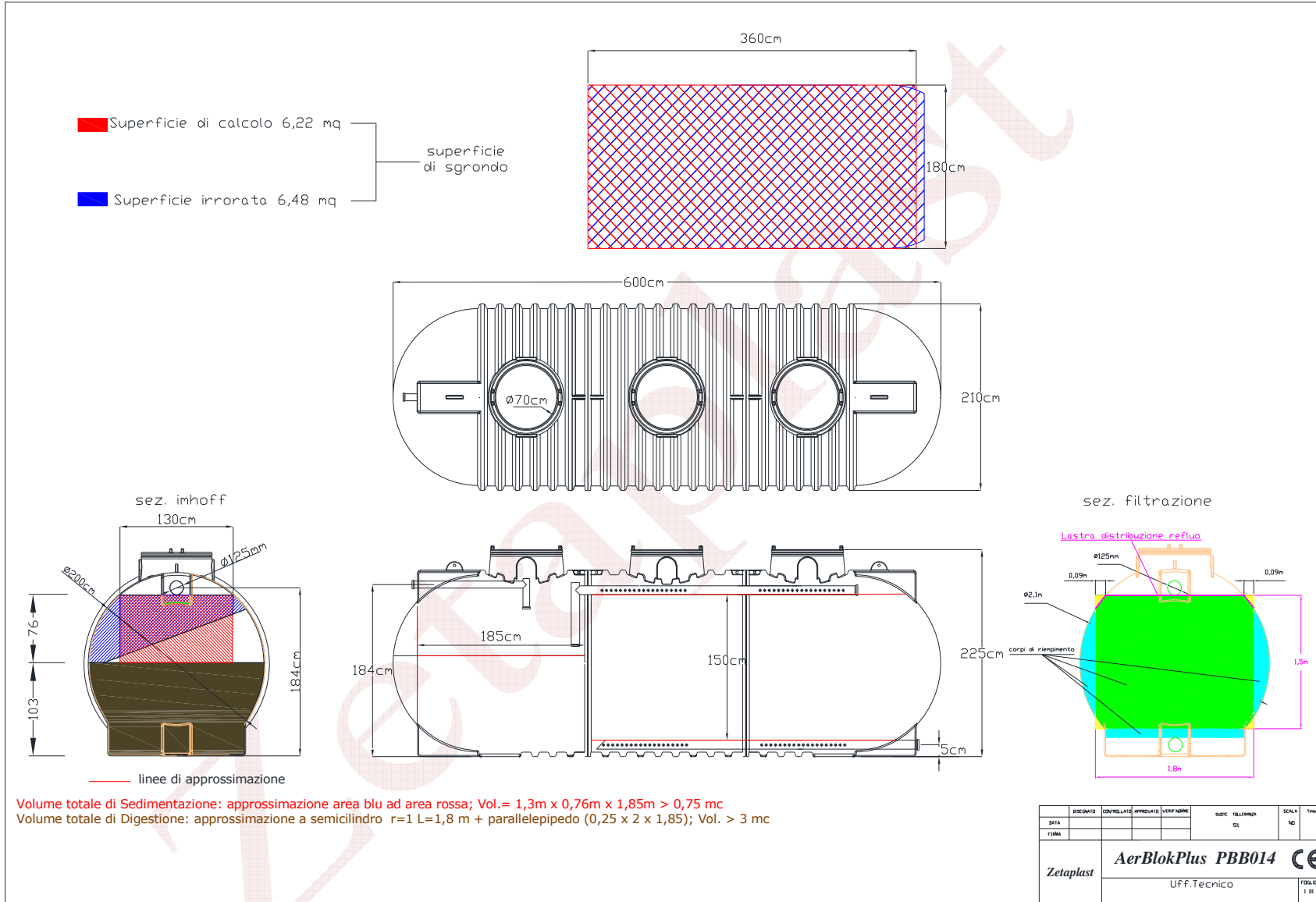
Fig.3 – Schema tecnico
