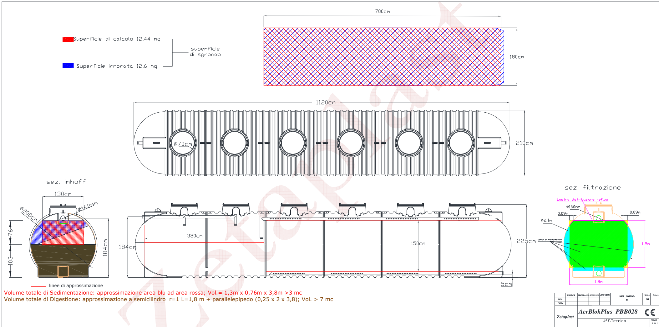
Fig.3 – Schema tecnica
