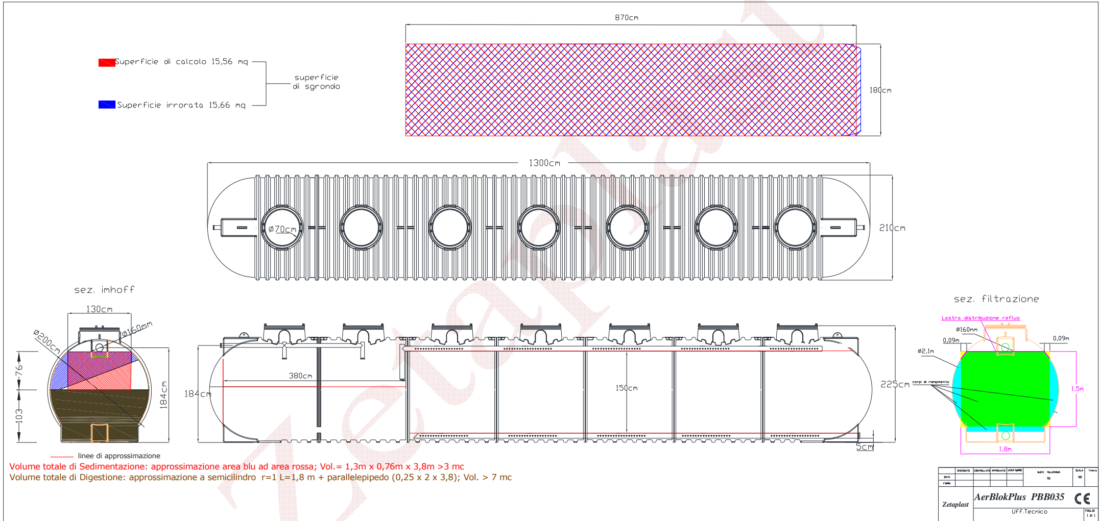
Fig.3 – Schema tecnico
