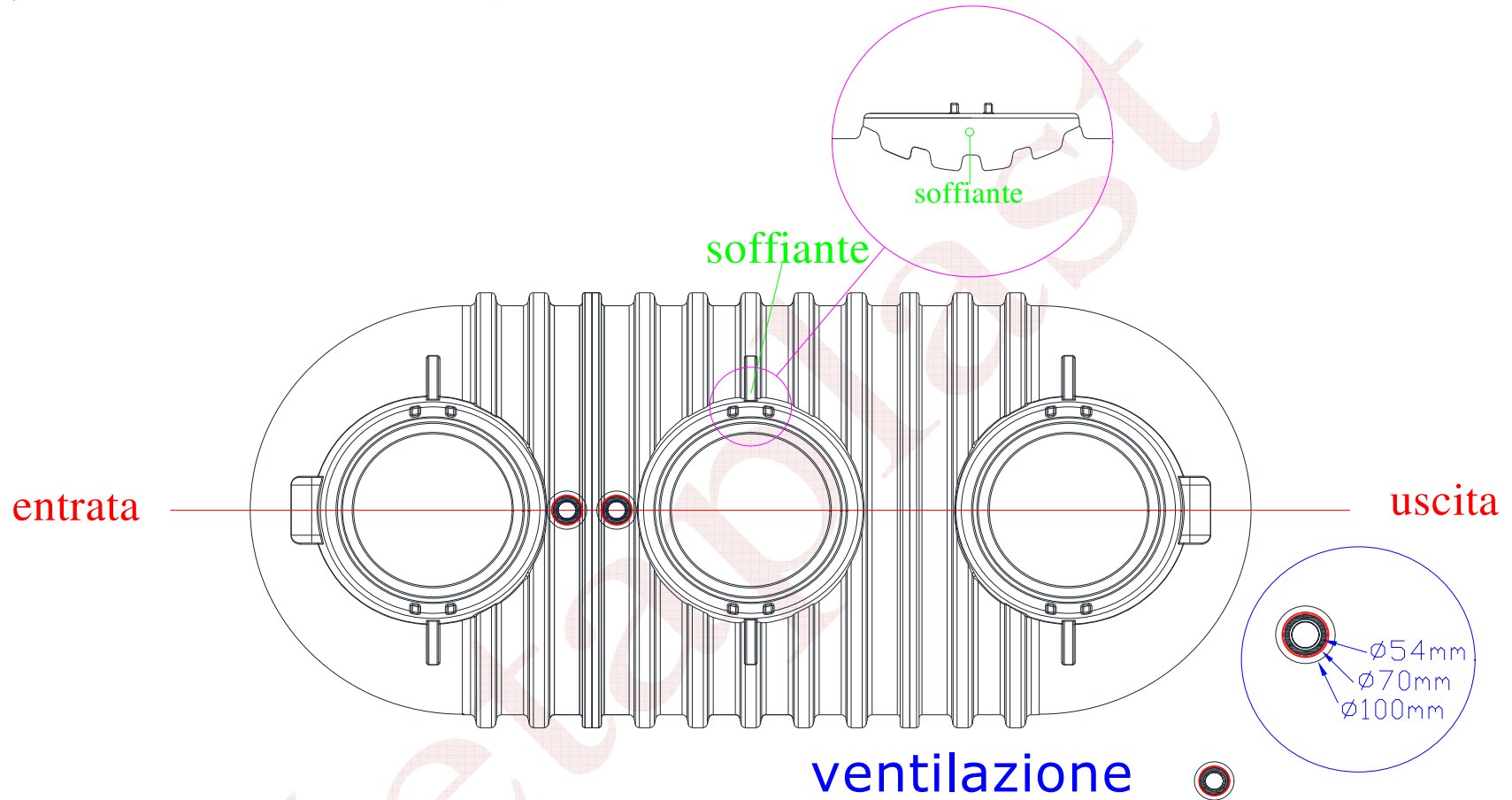
Fig.2 – Posizionamento collegamenti biogas
