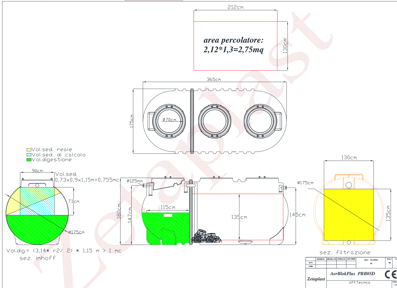
Fig.3 – Schema tecnica
