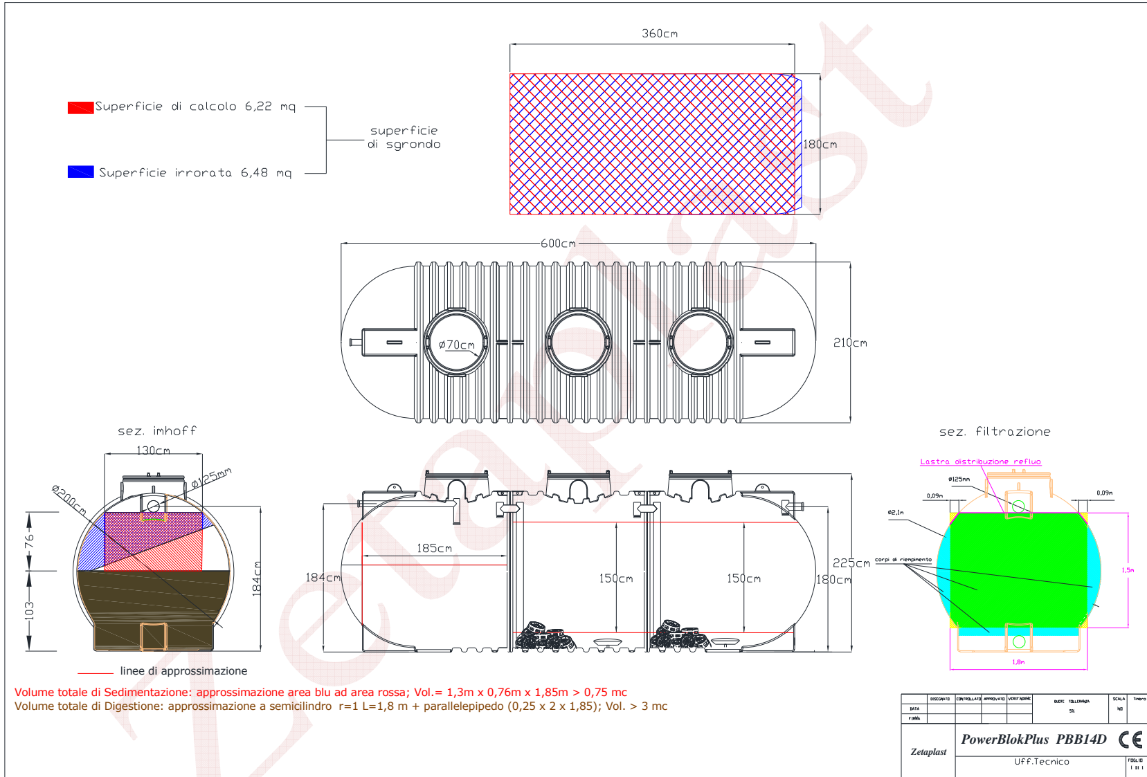
Fig.3 – Schema tecnica
