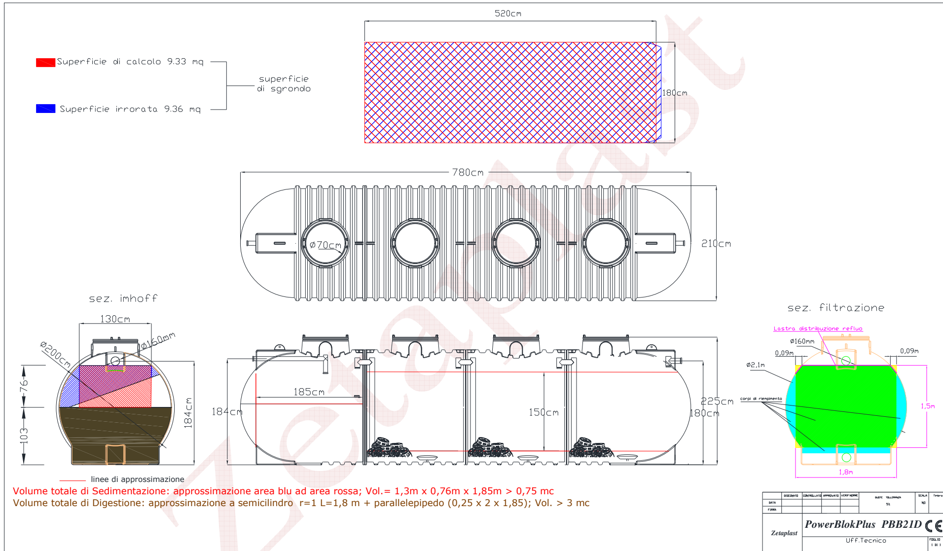
Fig.3 – Schema tecnica
