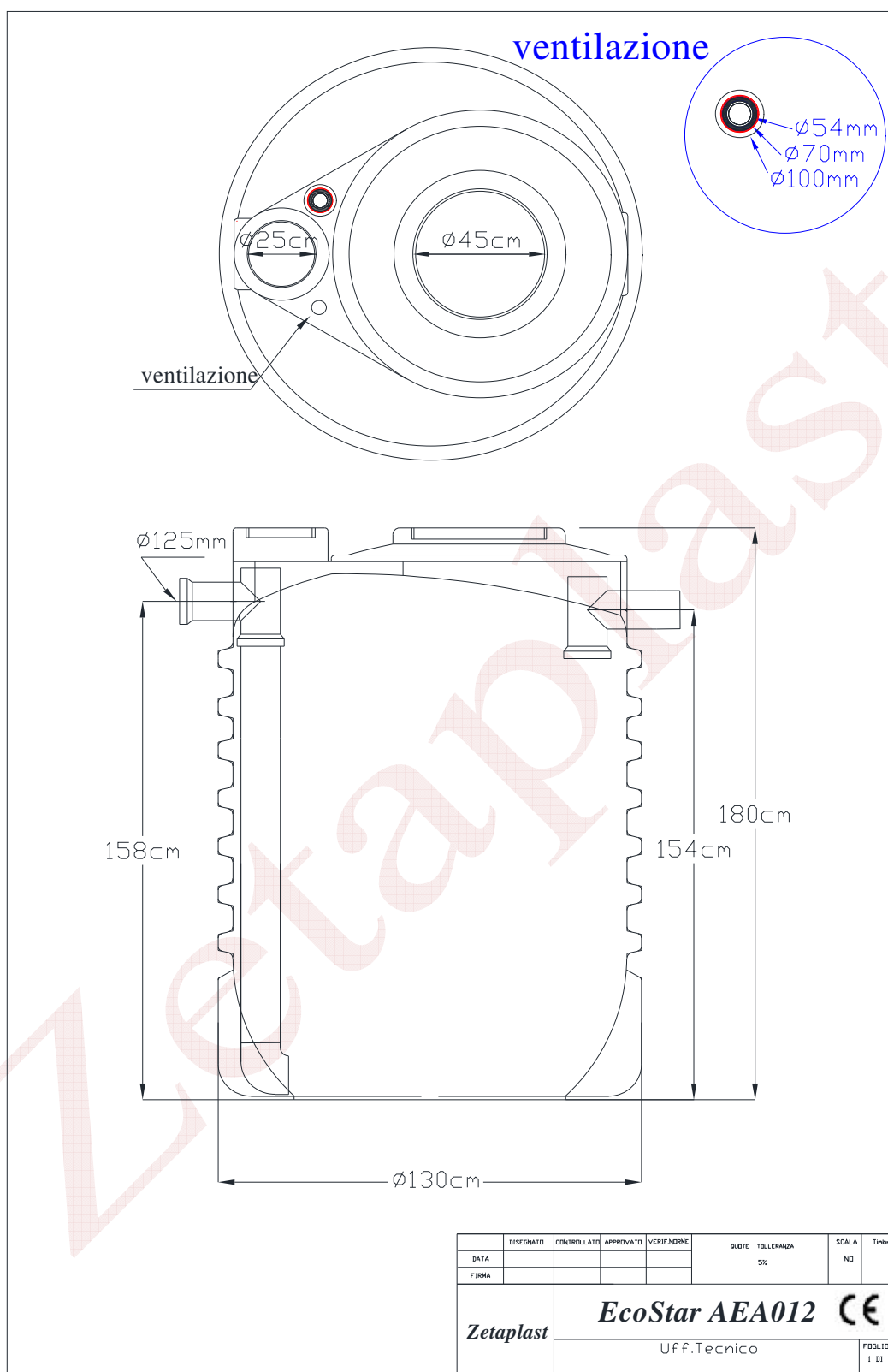
Fig.7 – Schema tecnico
