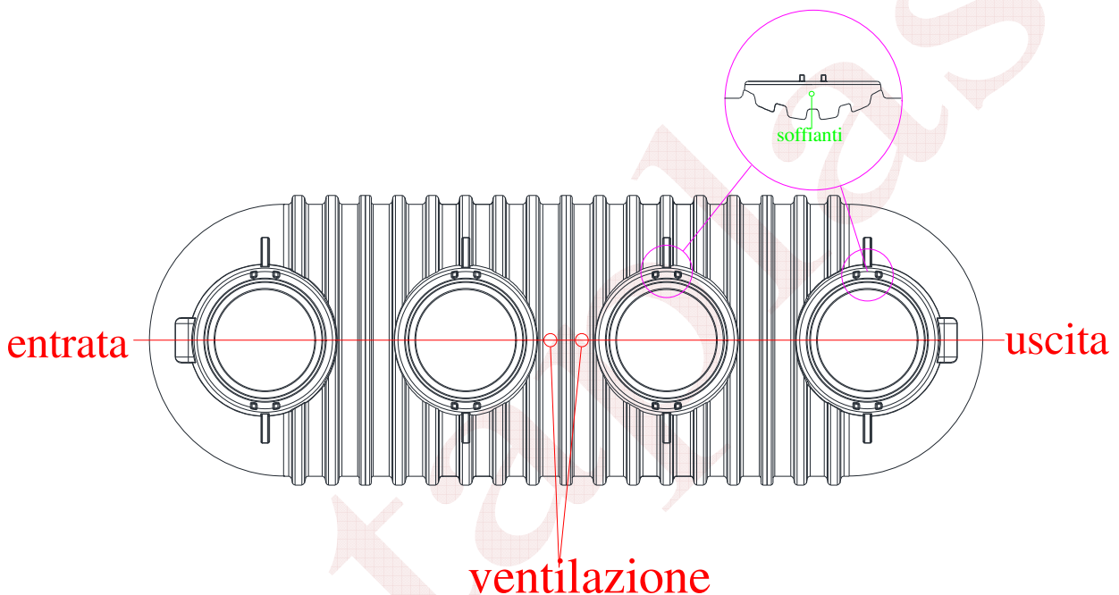
Fig.2 – Installazione sedimentatore
