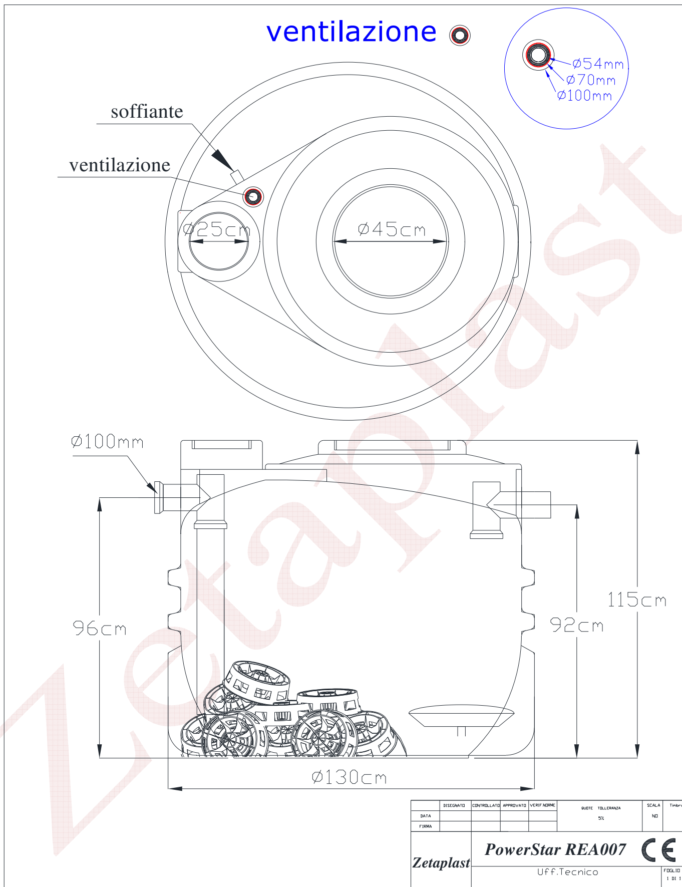
Fig.6 – Schema tecnico
