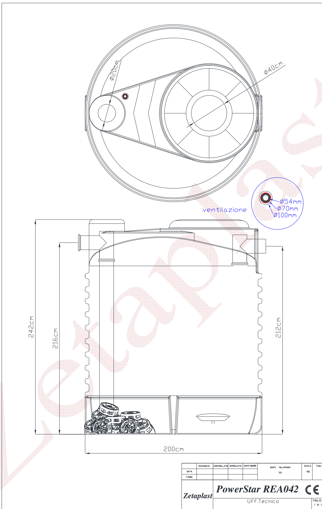
Fig.6 – Schema tecnico
