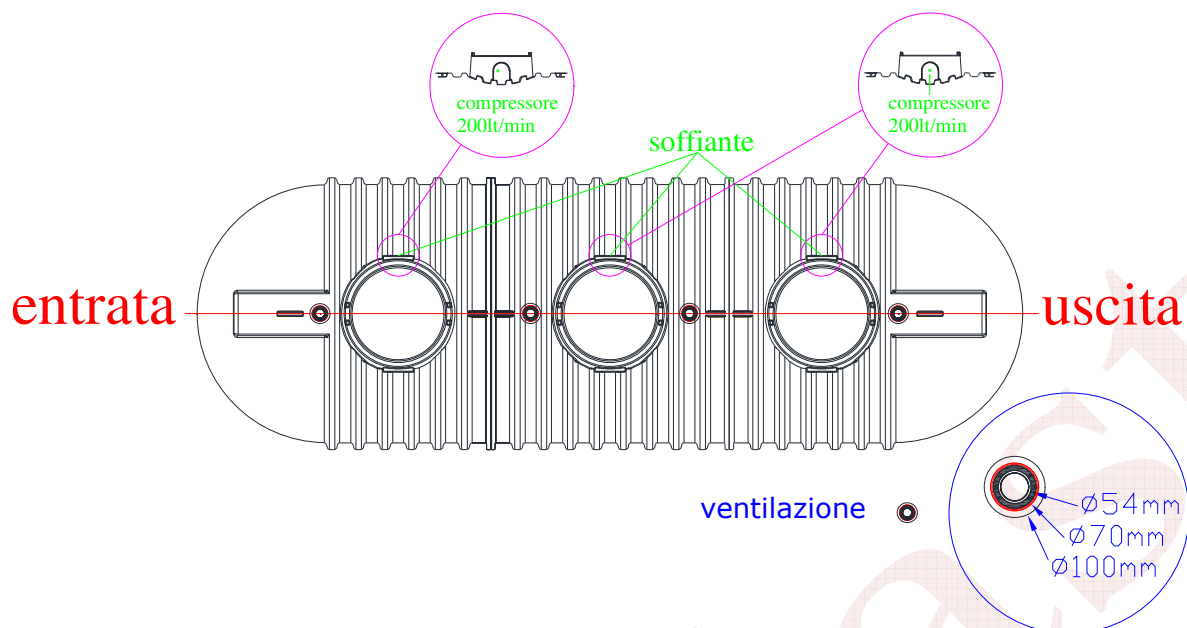
Fig.2 – Posizionamento collegamenti biogas e ossigenazione
