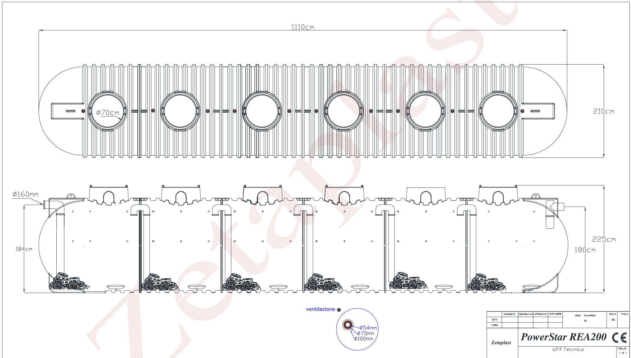
Fig.6 – Schema tecnico
