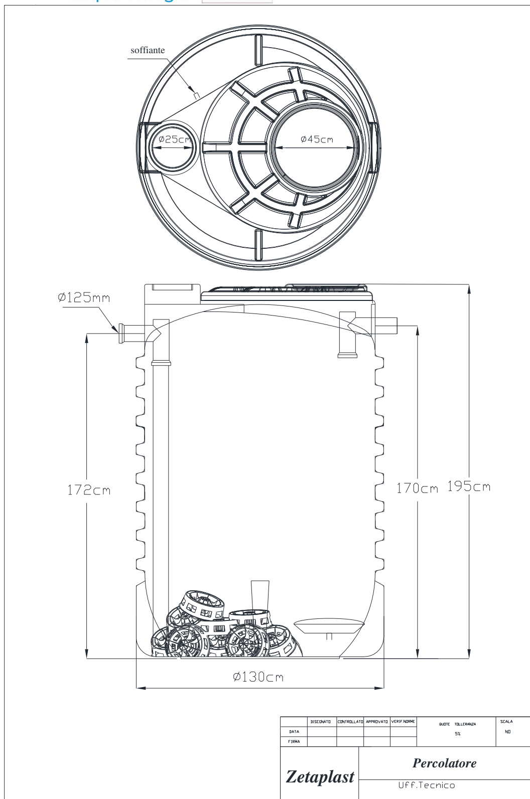
Fig.8 – Percolatore
