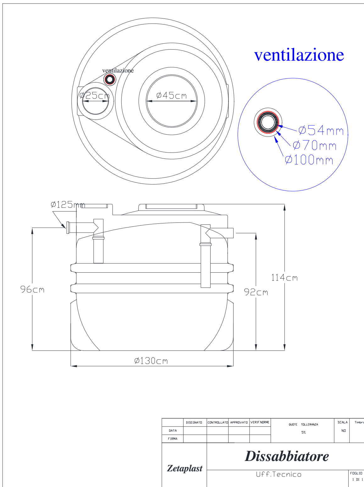
Fig.6 – Dissabbiatore
