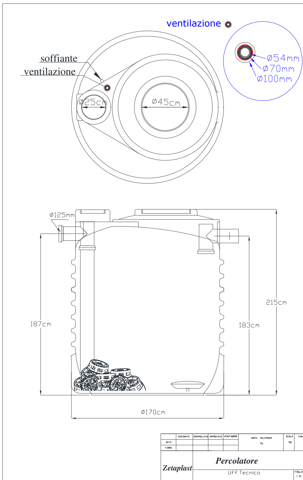
Fig.8 – Percolatore
