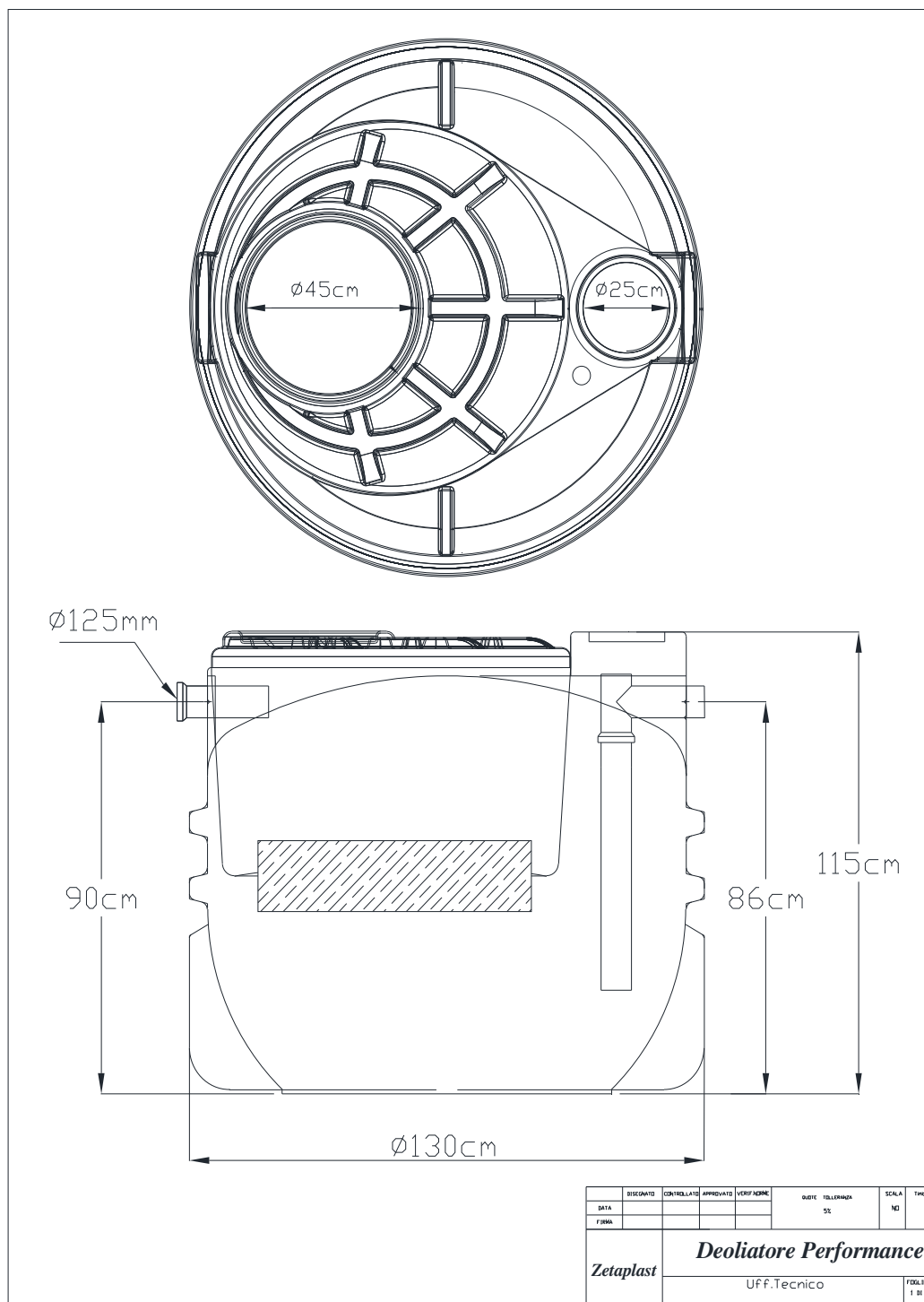
Fig.7 – Deoliatore
