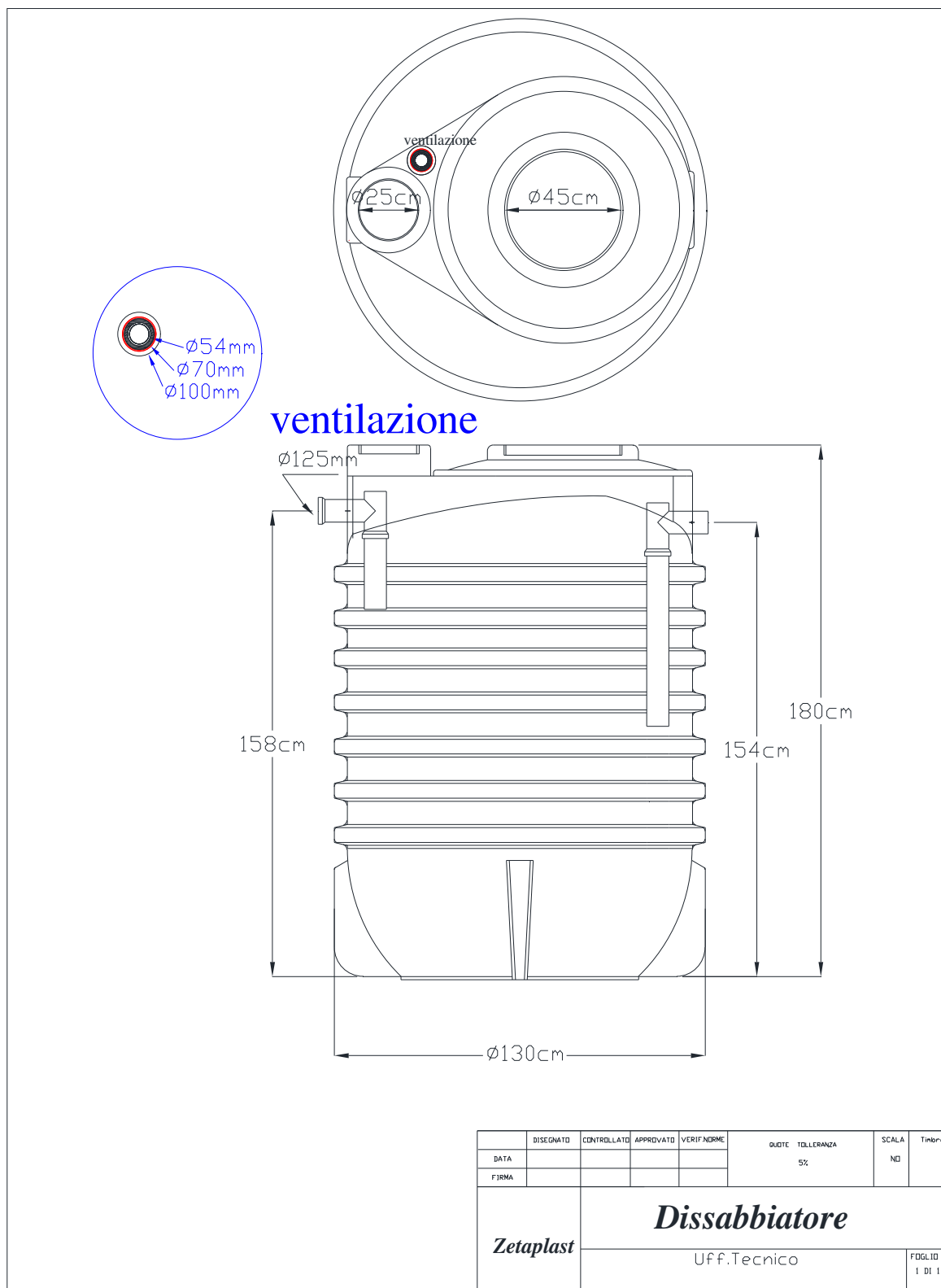
Fig.6 – Dissabbiatore
