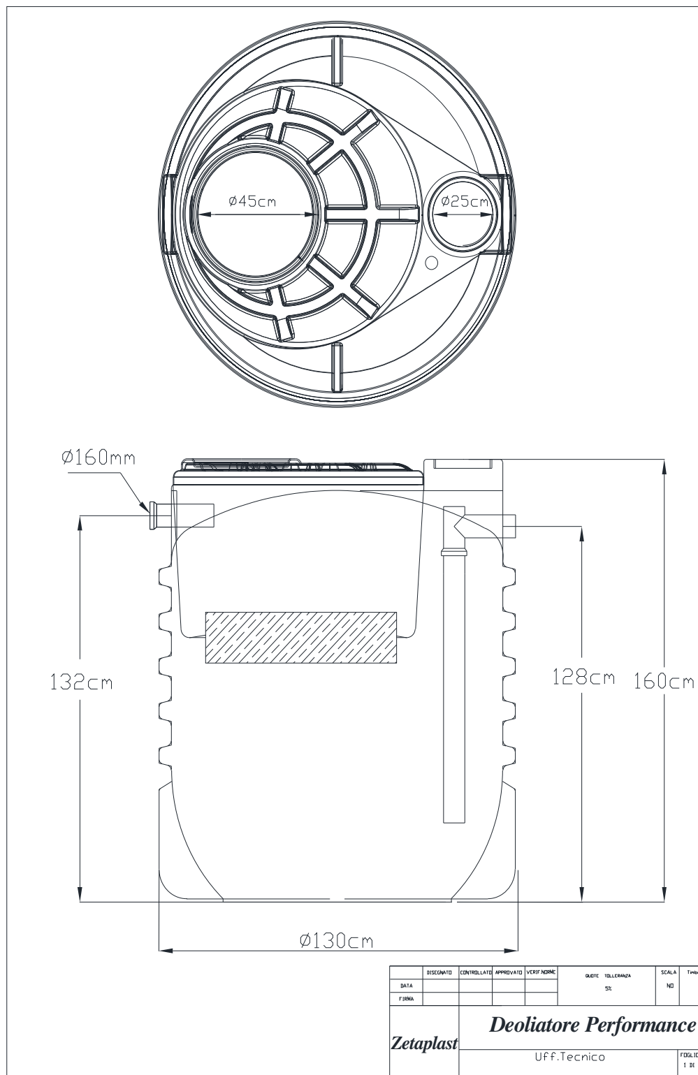
Fig.7 – Deoliatore
