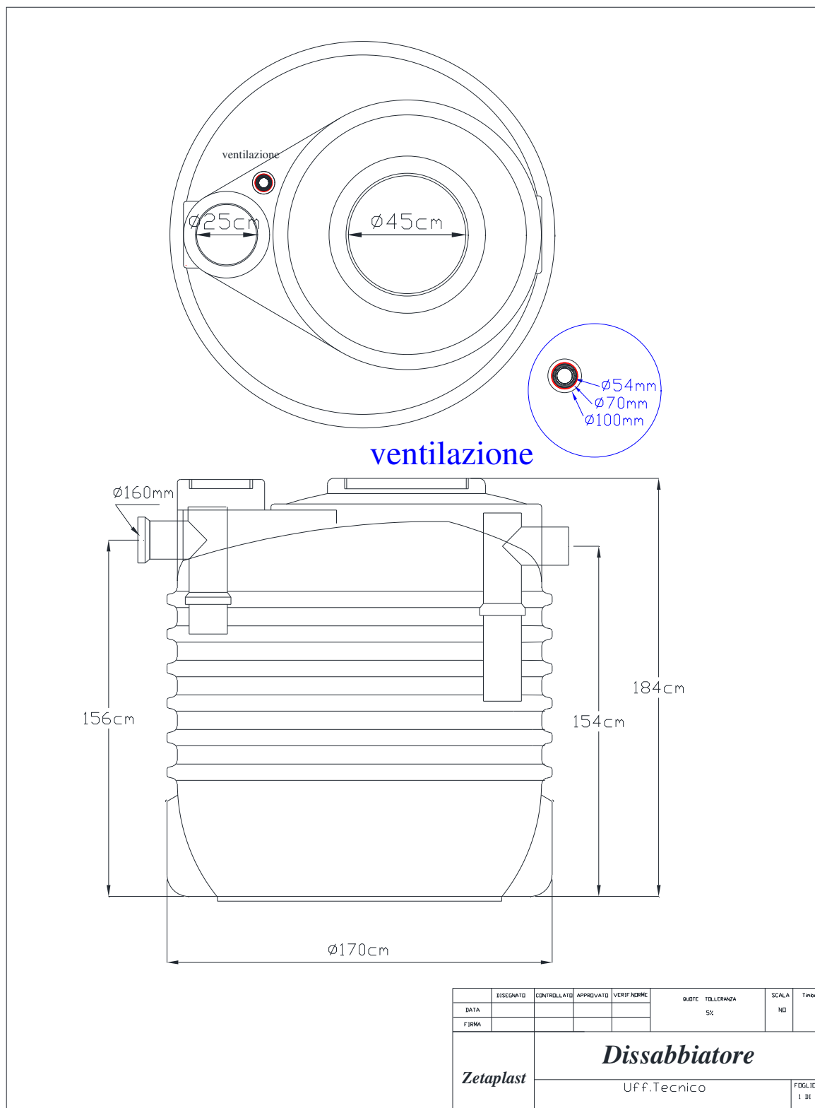
Fig.6 – Dissabbiatore
