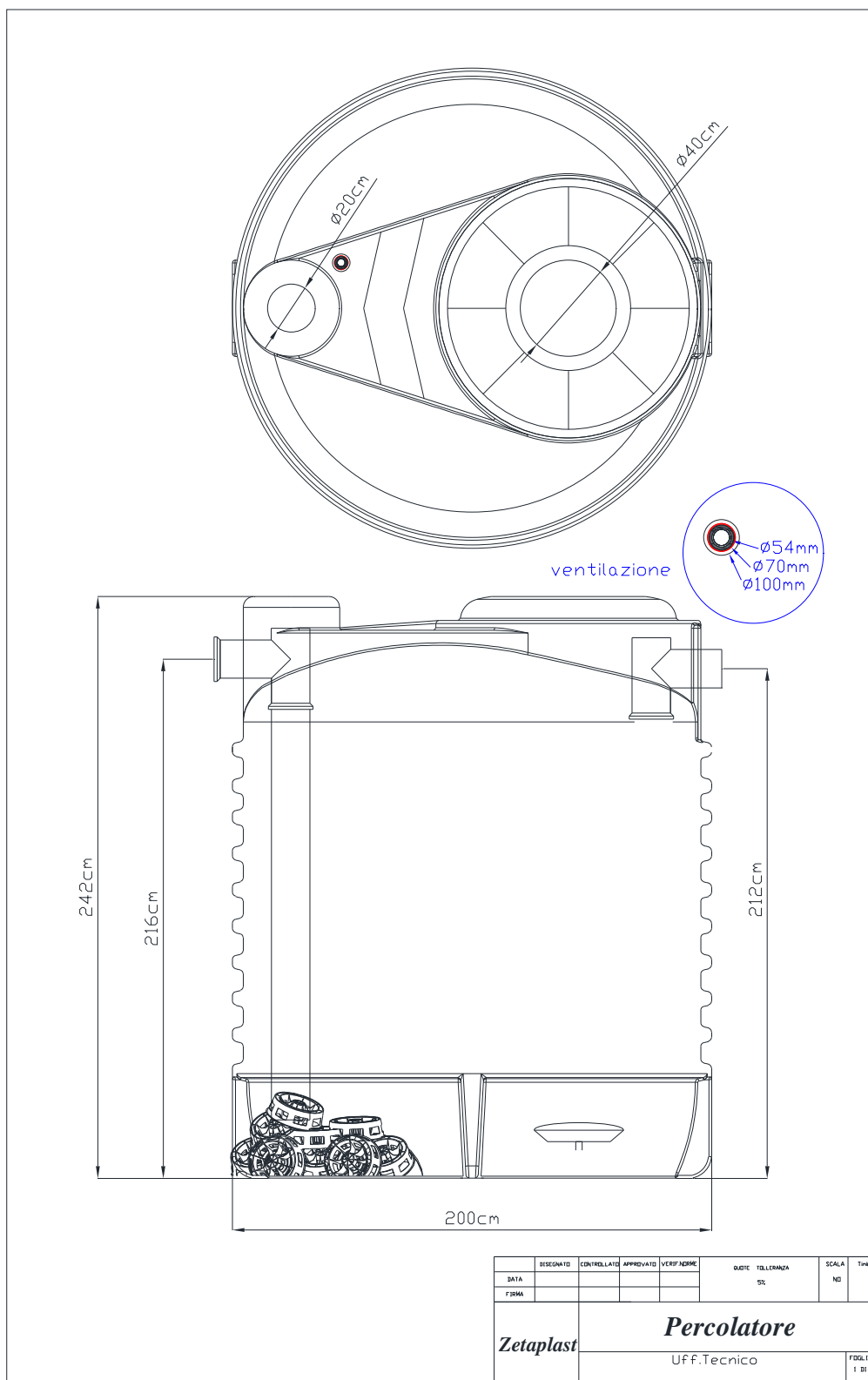
Fig.8 – Percolatore
