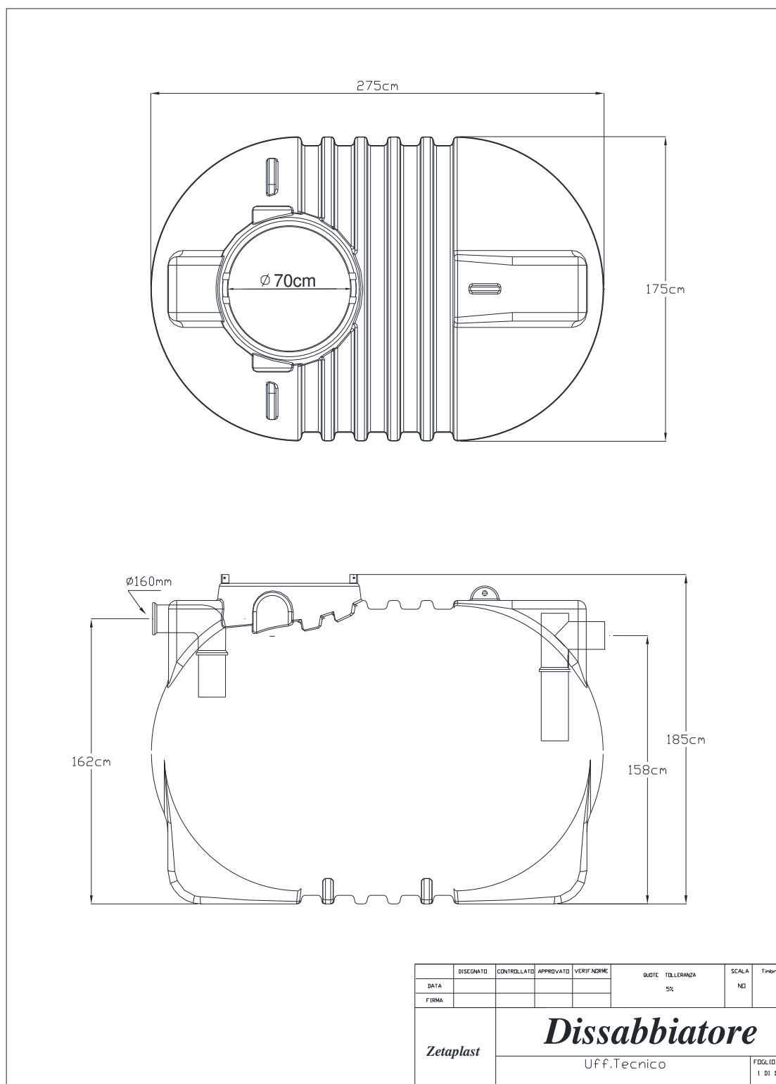
Fig.6 – Dissabbiatore
