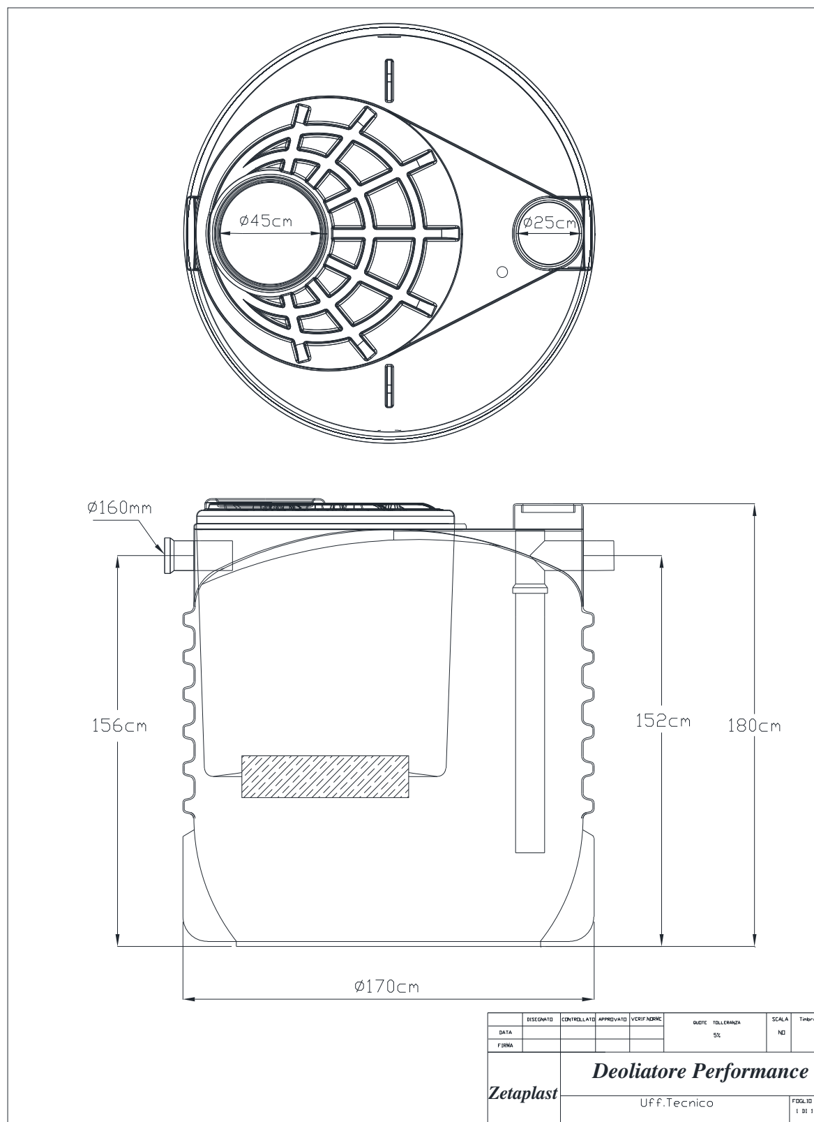
Fig.7 – Deoliatore
