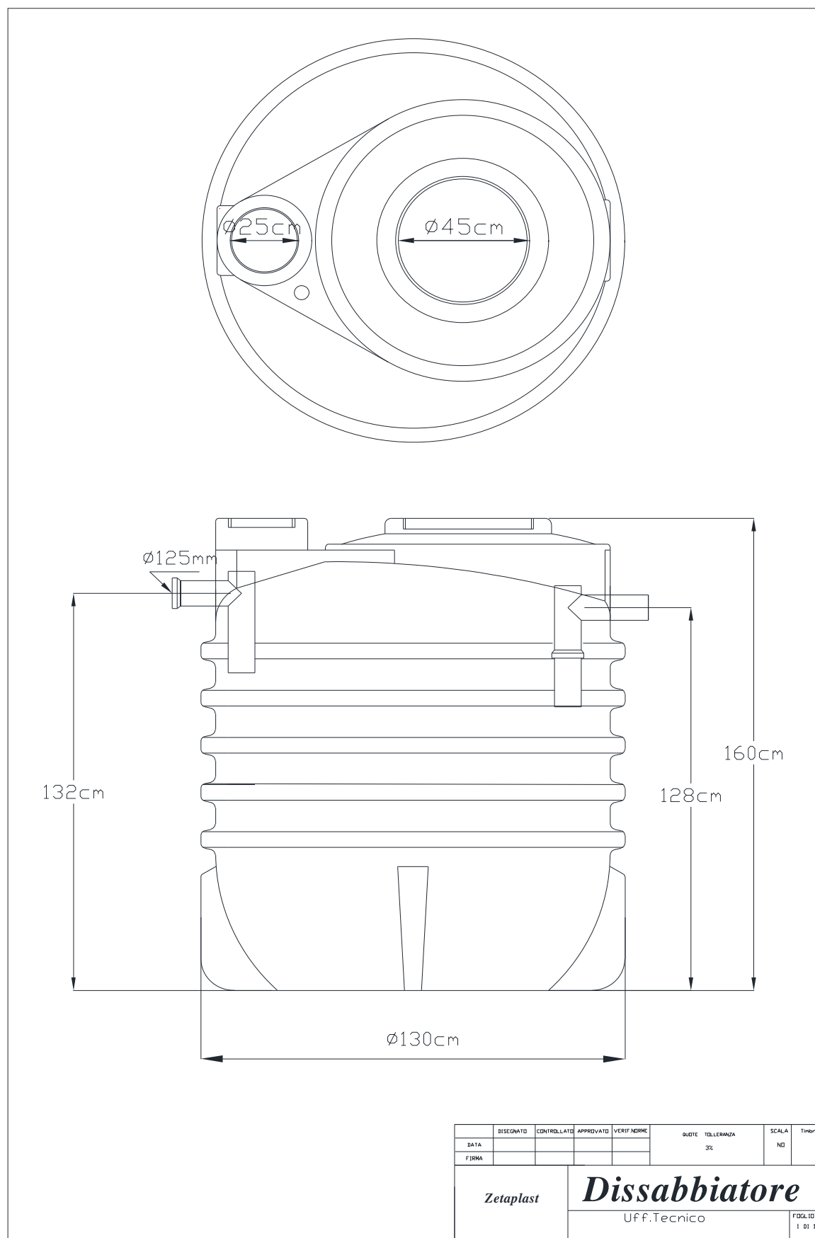
Fig.7 – Dissabbiatore
