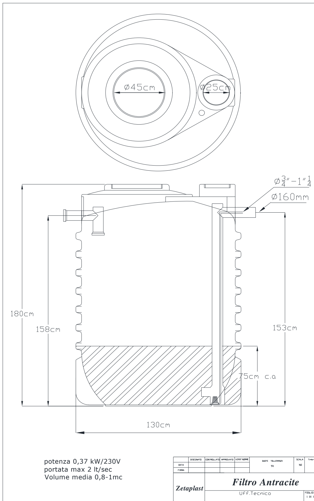
Fig.10 – Filtro Antracite
