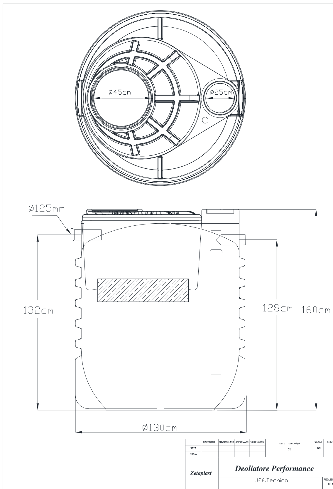
Fig.8 – Deoliatore
