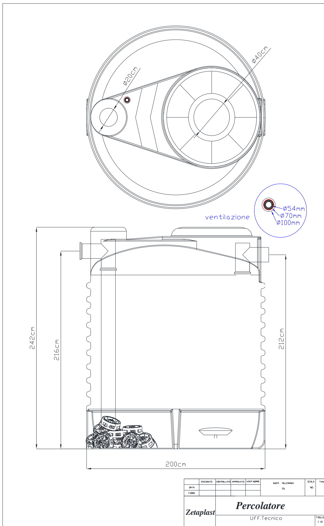
Fig.9 – Percolatore
