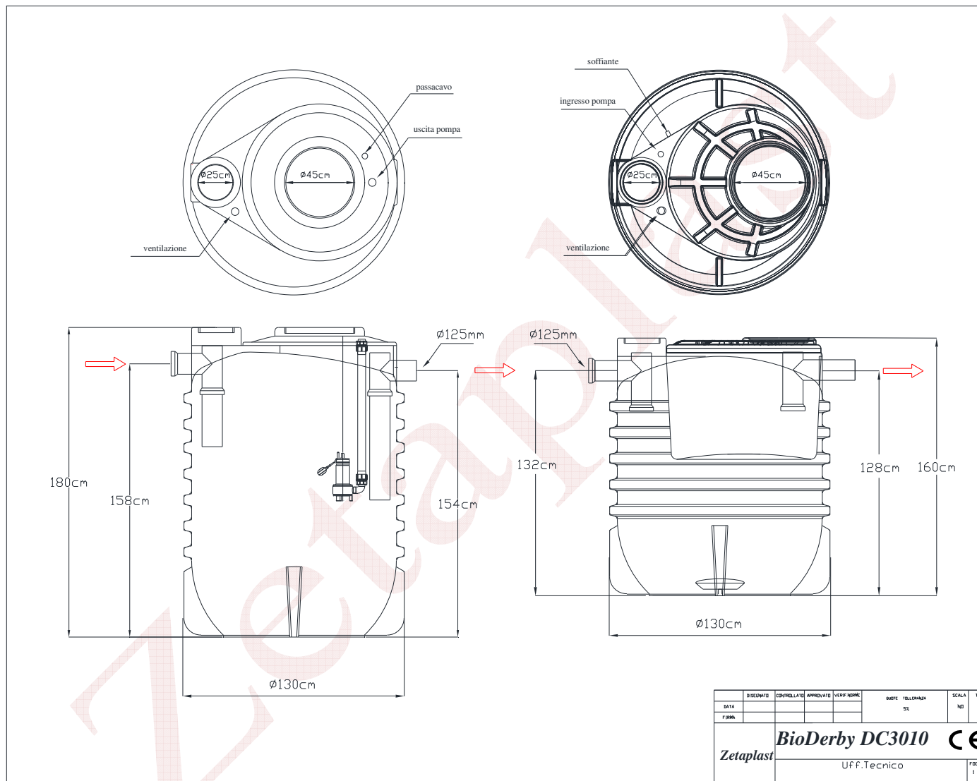
Fig.3 – Schema tecnico
