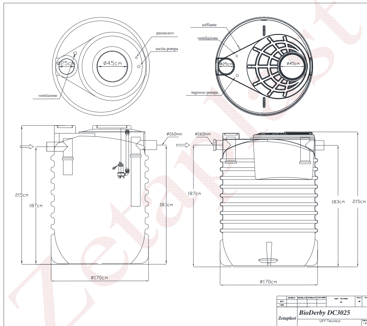
Fig.3 – Schema tecnico
