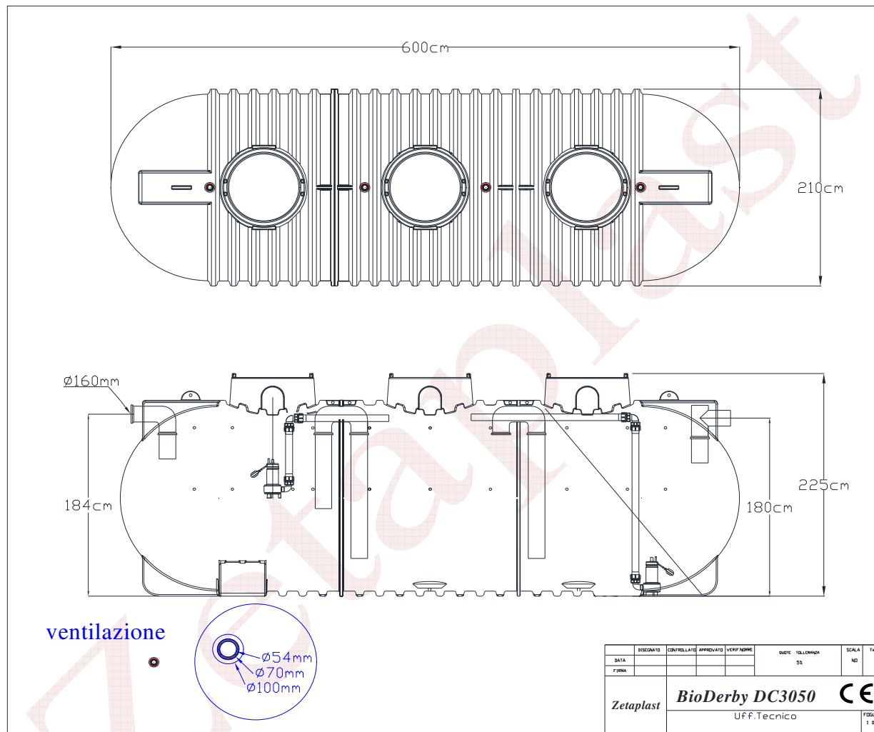
Fig.7 – Schema tecnico
