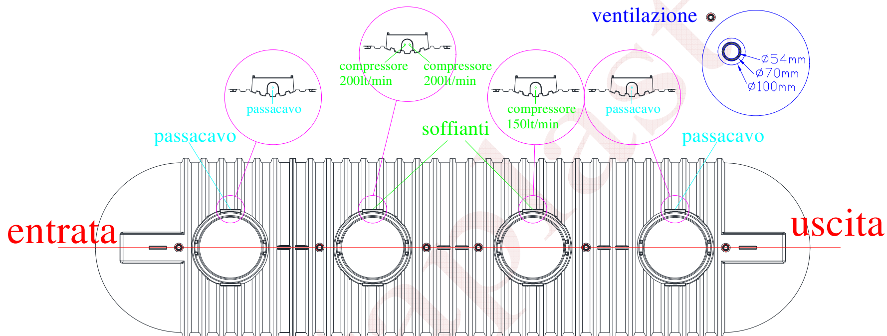
Fig.2 – Posizionamento collegamenti biogas, ossigenazione e pompa
