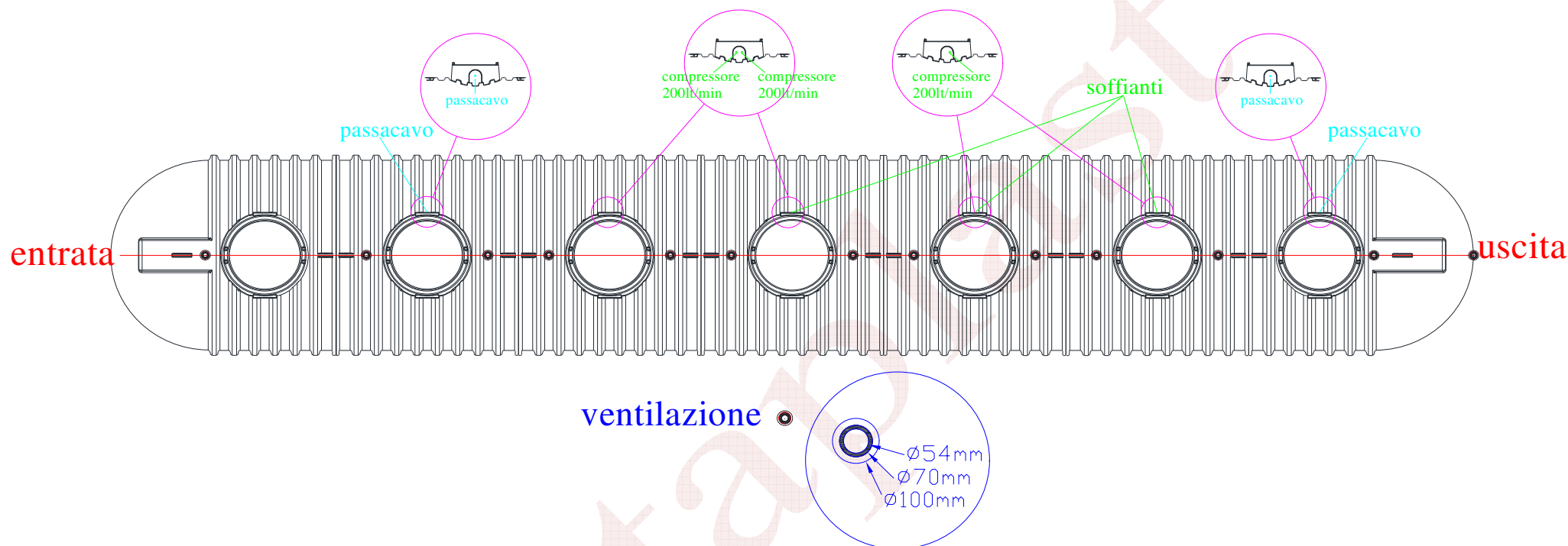
Fig.2 – Posizionamento collegamenti biogas, ossigenazione e pompa
