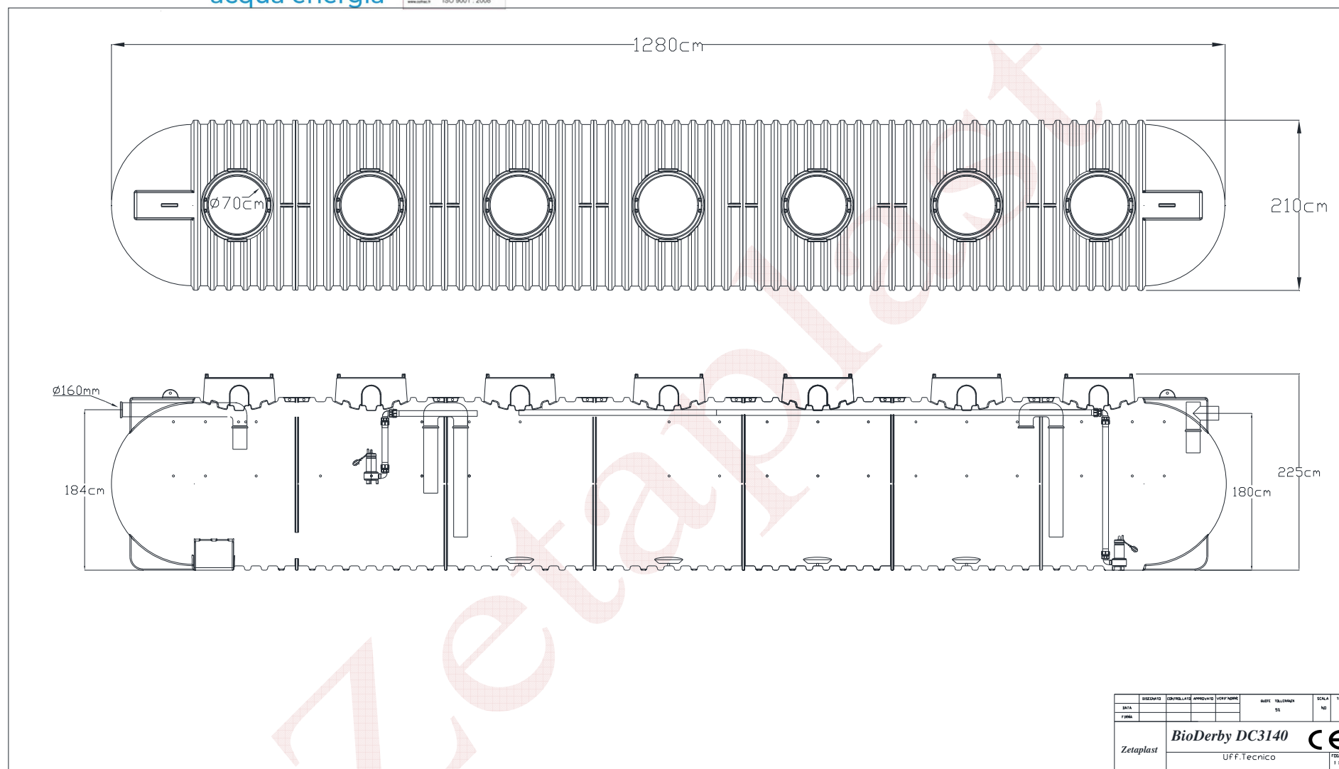
Fig.7 – Schema tecnico
