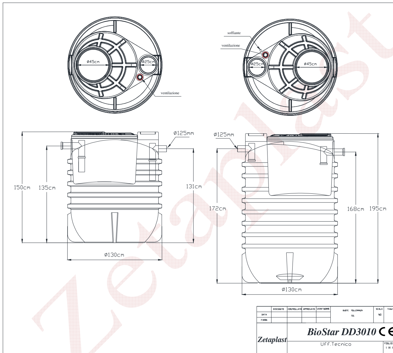
Fig.6 – Schema tecnico
