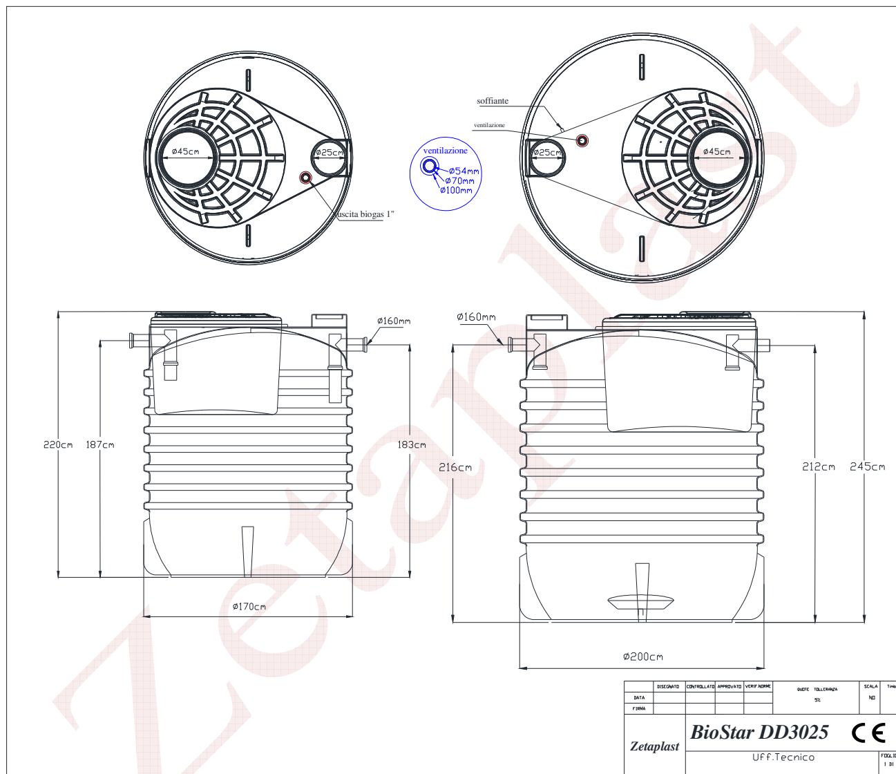
Fig.6 – Schema tecnico
