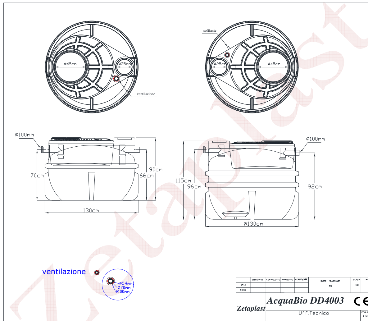
Fig.6 – Schema tecnico
