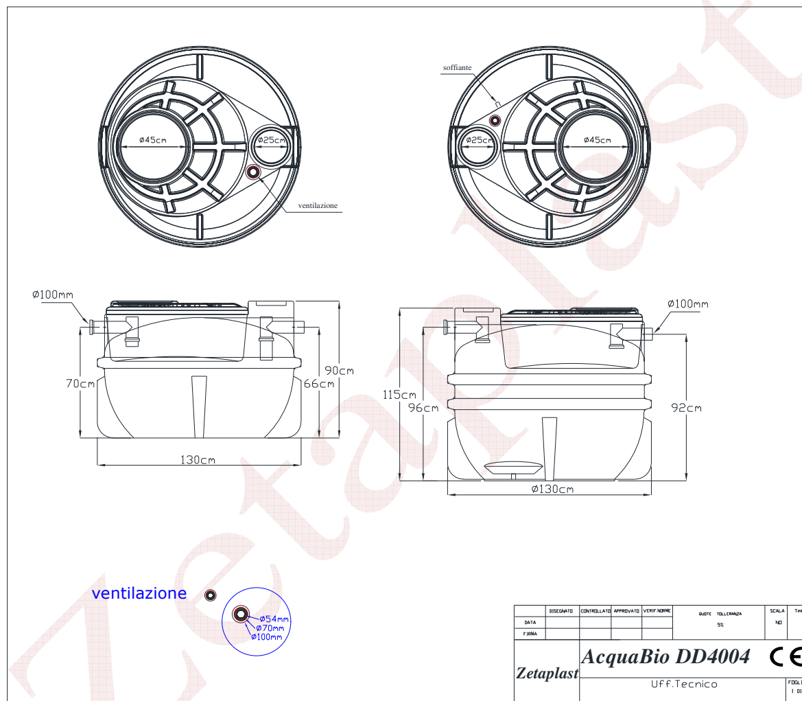
Fig.6 – Schema tecnico
